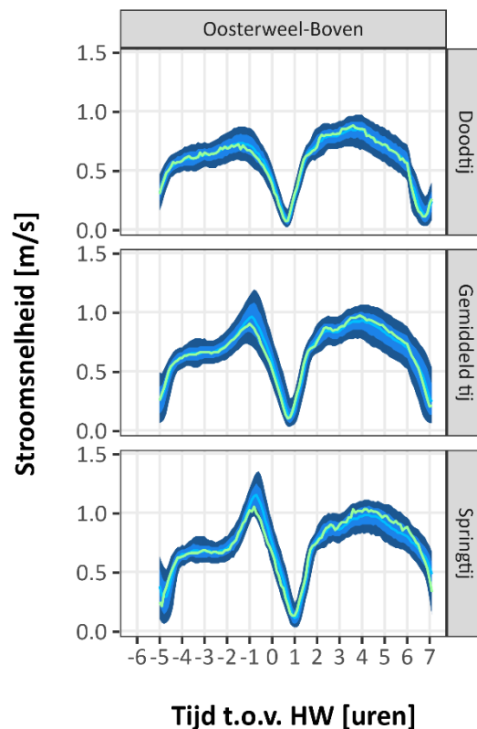
Figuur 37 – Historische vergelijking van 2023 van de stroomsnelheid over een getijcyclus (ensemble analyse) voor doodtij, gemiddeld tij en springtij ter hoogte van Oosterweel (data vanaf 2001). Relatieve tijd is t.o.v. HW in Antwerpen.
