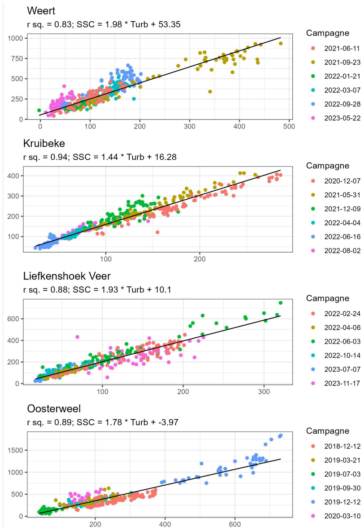
Figuur 106 – De SSC-turbiditeitsrelaties voor Liefkenshoek Veer, Oosterweel, Kruikeke en Weert,
