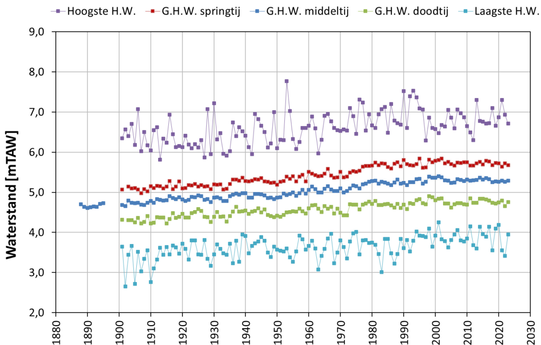
Figuur 12 – Antwerpen-Loodsgebouw: langjarige tij-evolutie (1888-2023) van jaargemiddeld hoogwater middeltij, springtij en doottij, aangevuld met de jaarlijks hoogste en de jaarlijks laagste hoogwaterstanden.
