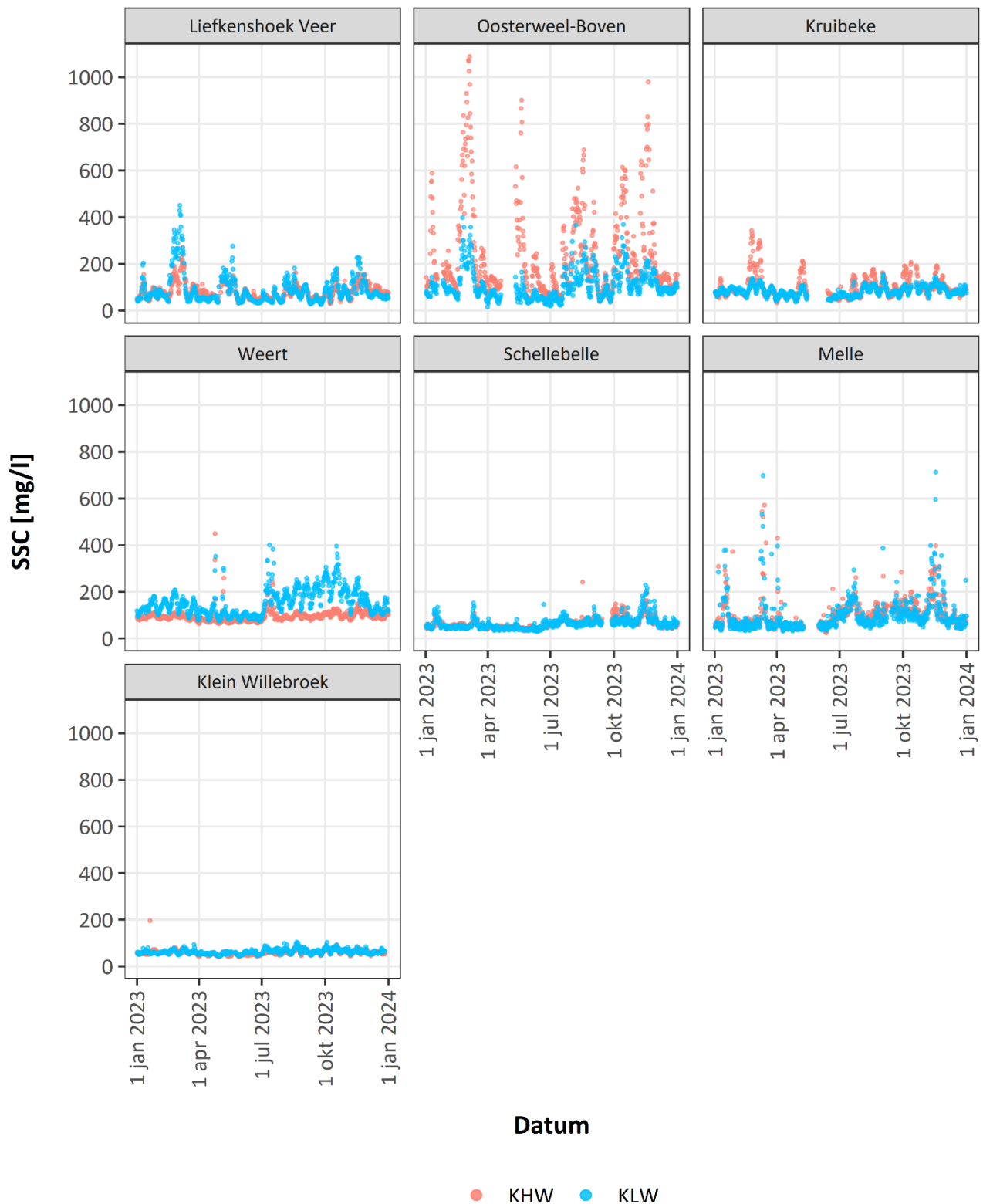
Figuur 52 – SSC (gemiddelde) verloop in 2023 tijdens eb enloed voor de verschillende meetstations.
