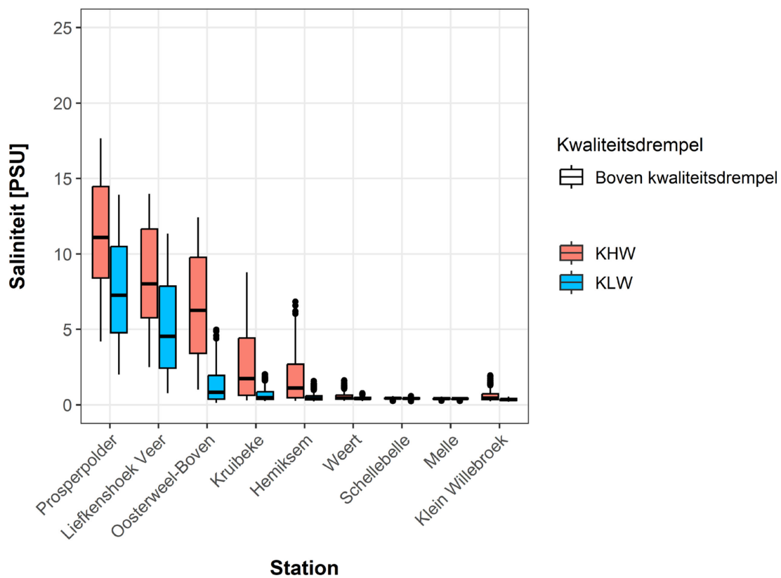
Figuur 47 – Jaarstatistieken (2023) voor saliniteit KHW max en KWL min voor de verschillende meetstations.
