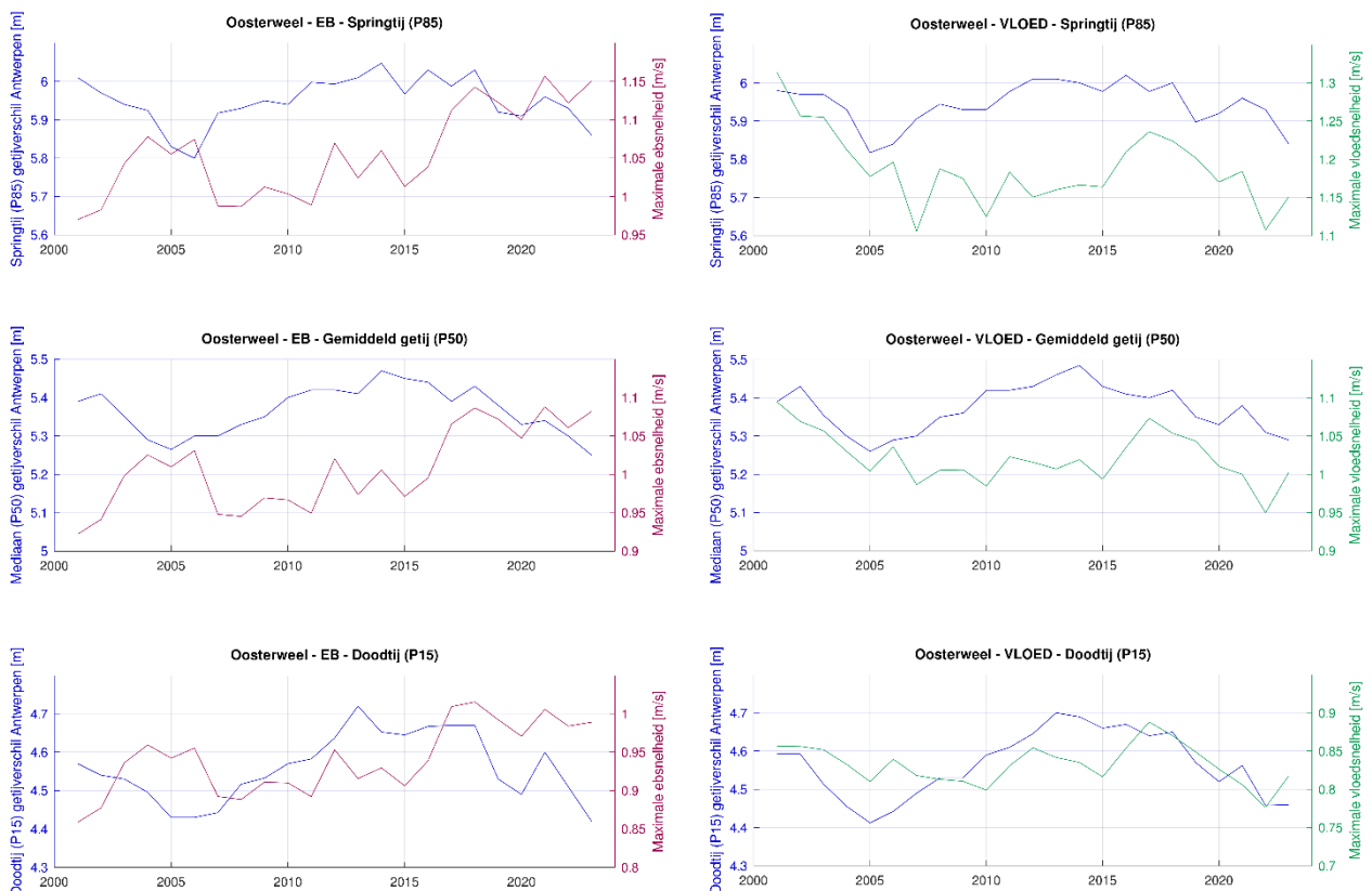
Figuur 40 – Verloop van het getijverschil en de maximale stroomsnelheid tijdens eb en vloed bij springtij, gemiddeld tij en doodtij
