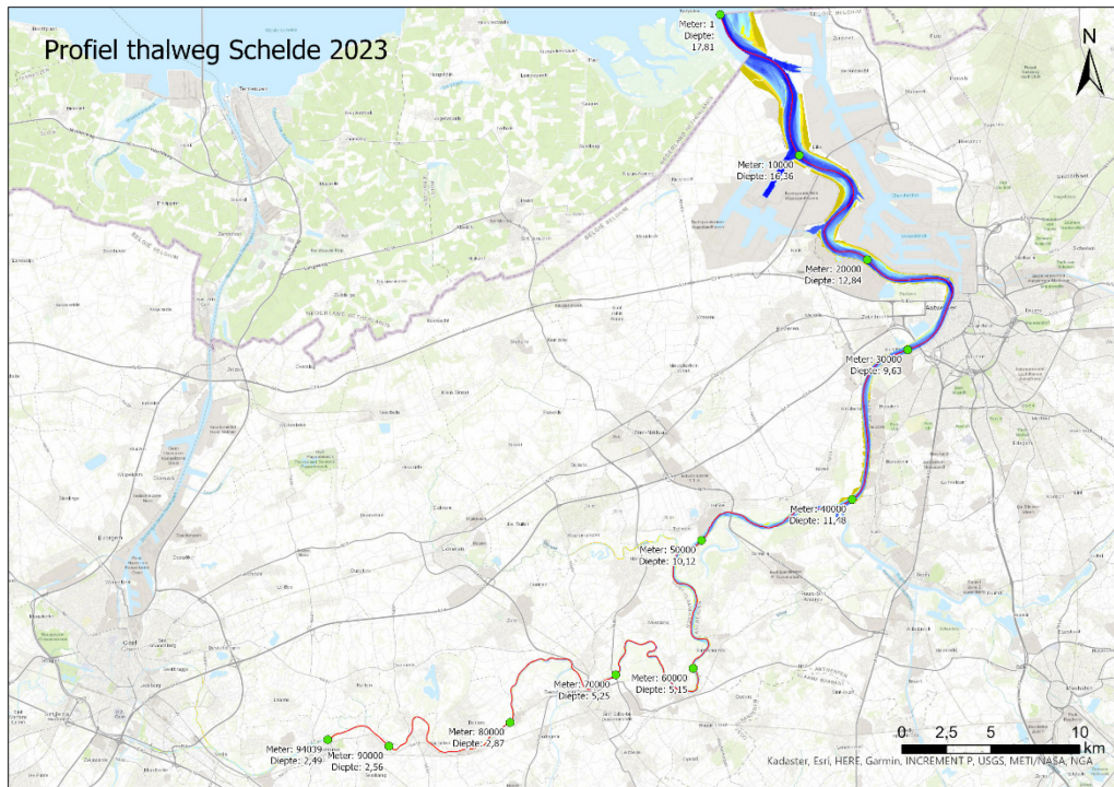
Figuur 83 – Ligging langsprofiel Zeeschelde
