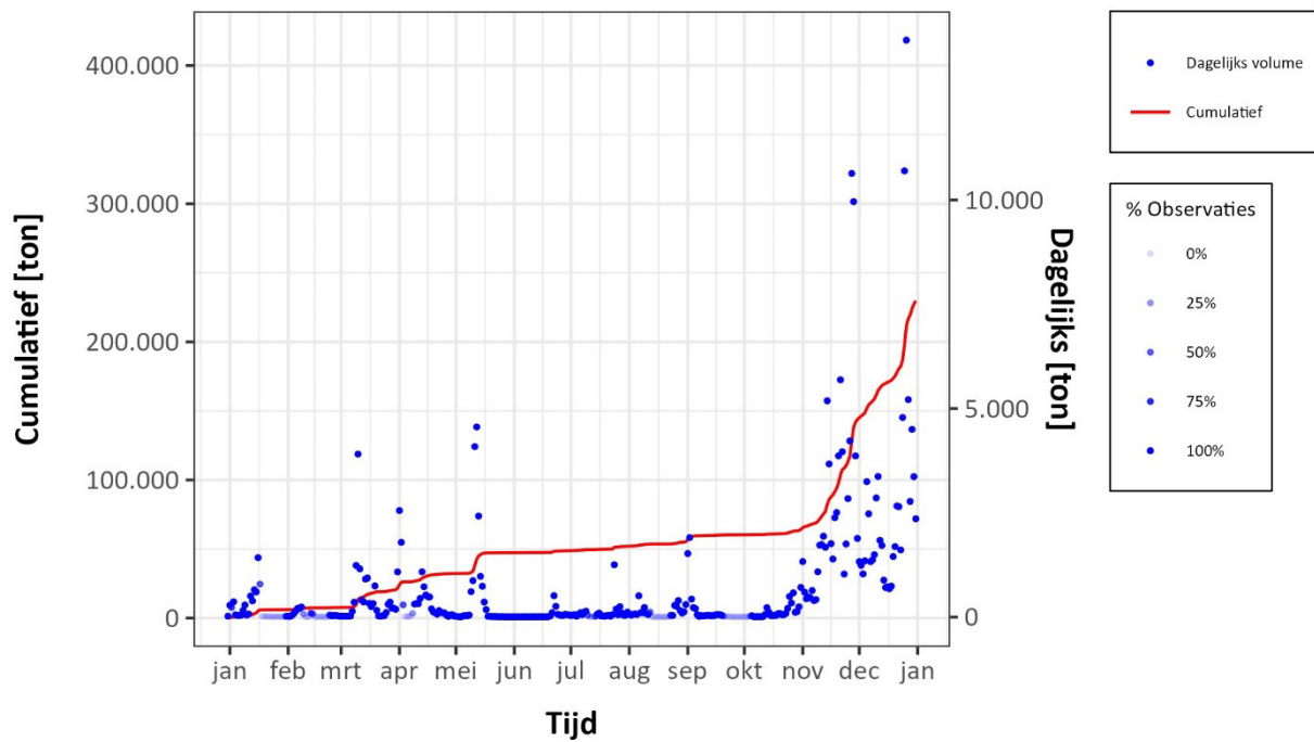
Figuur 78 – Berekende dagelijkse en gecumuleerde sedimentvracht in Eppegem komende van de Zenne (EWI-correctie toegepast).
