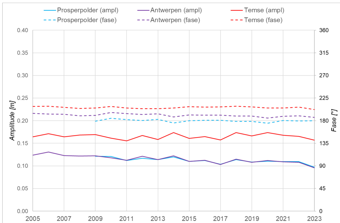
Figuur 103 – Evolutie in de tijd van de amplitude en fase van de M4-component (afwaartse posten)
