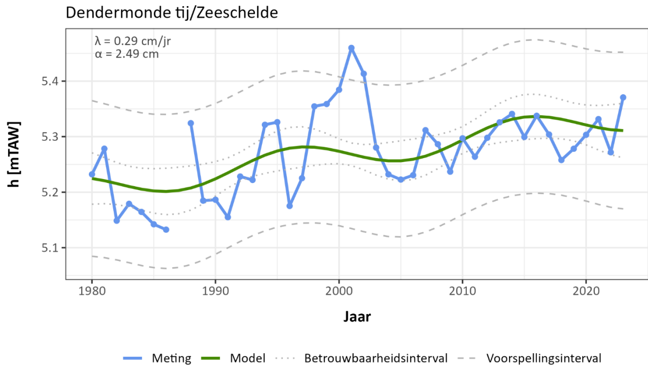
Figuur 97 – Trend jaargemiddeld hoogwater te Dendermonde bepaald over de periode 1980-2023.
