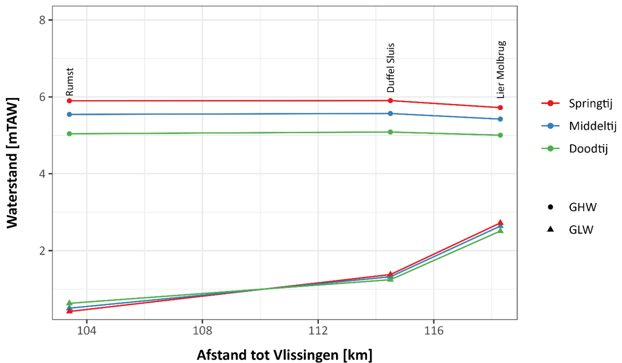
Figuur 5 – Gemiddeld hoogwater (GHW) en gemiddeld laagwater (GLW) bij middeltij, springtij en doottij in 2023 voor de Beneden-Nete.
