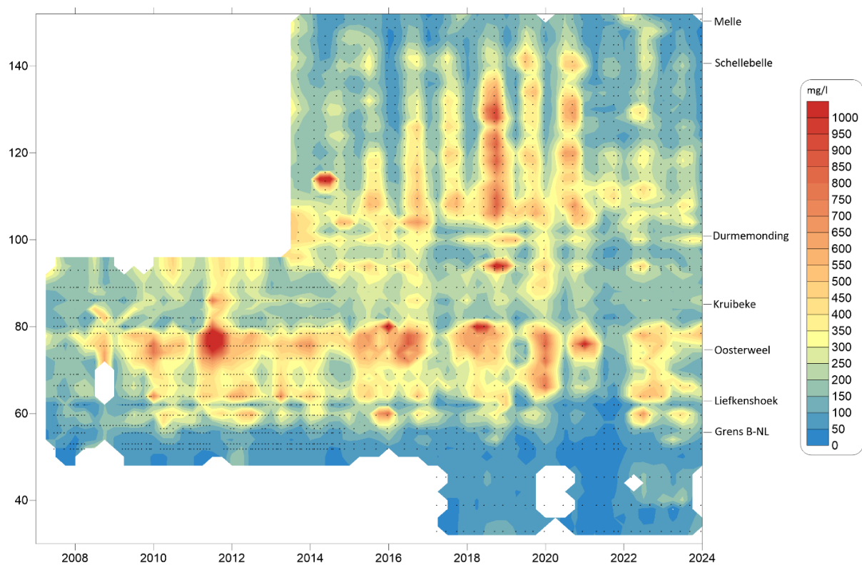
Figuur 67 – Sedimentconcentratie nabij de bodem (mg/l) bij halftij-eb langs de Zeeschelde (interpolatietechniek: Kriging, zoekradius X-as: 0,25 jaar, zoekradius Y-as: 2 km)
