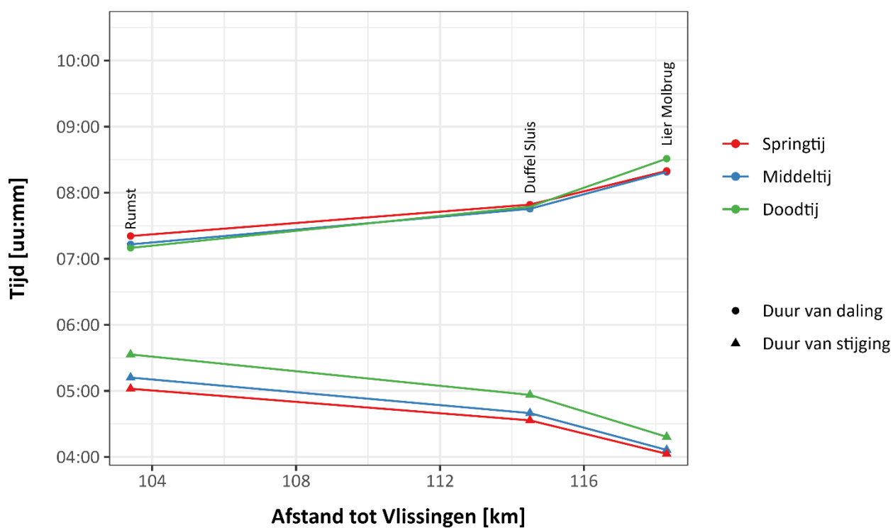
Figuur 7 – Duur van stijging en daling bij middeltij, springtij en doodtij in 2023 voor de Beneden-Nete.
