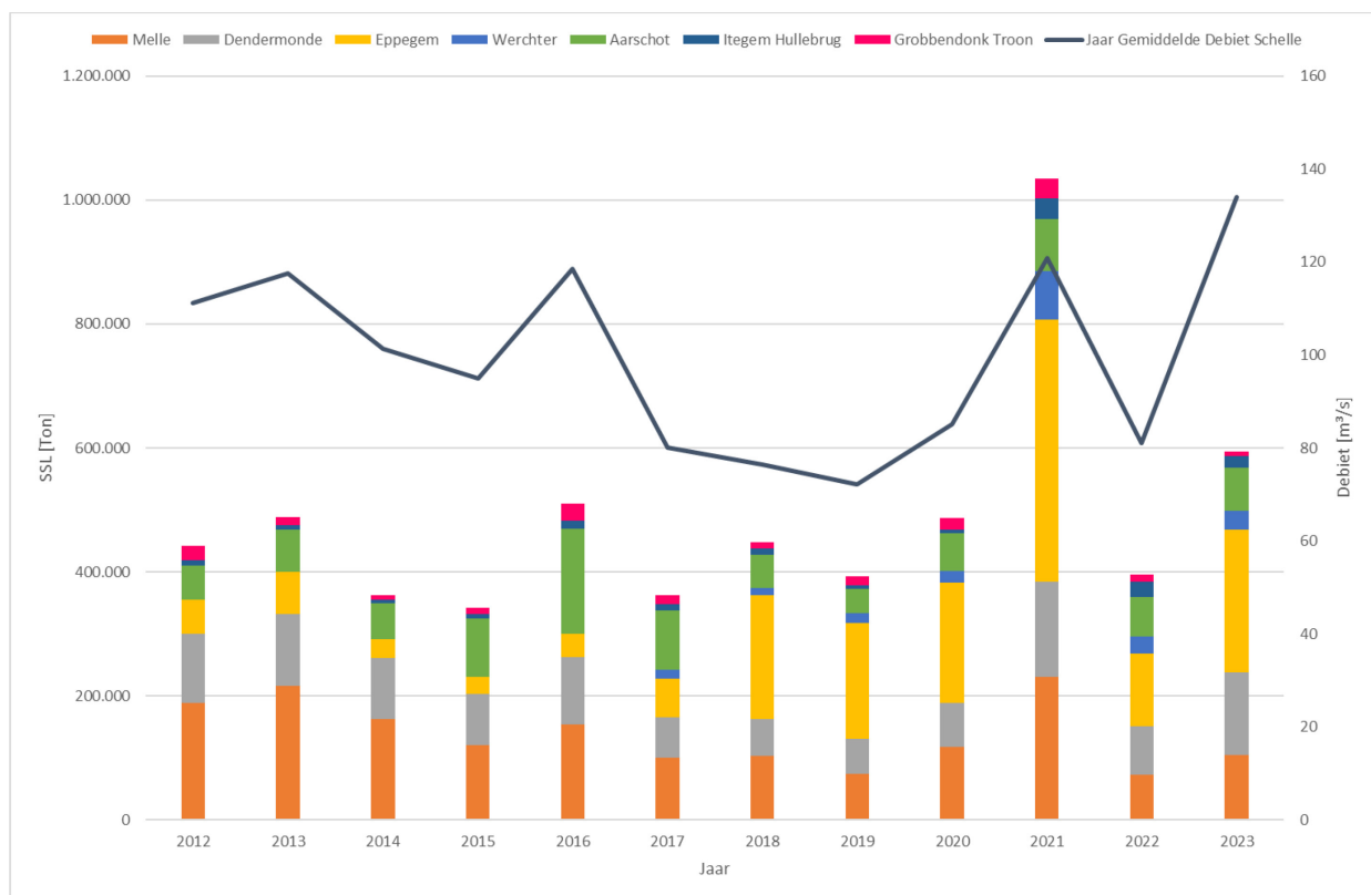
Figuur 75 – Historisch overzicht van de sedimentvrachten per stroomgebied (EWI-gecorrigeerd). Voor de locatie Werchter is pas data beschikbaar vanaf 2017.
