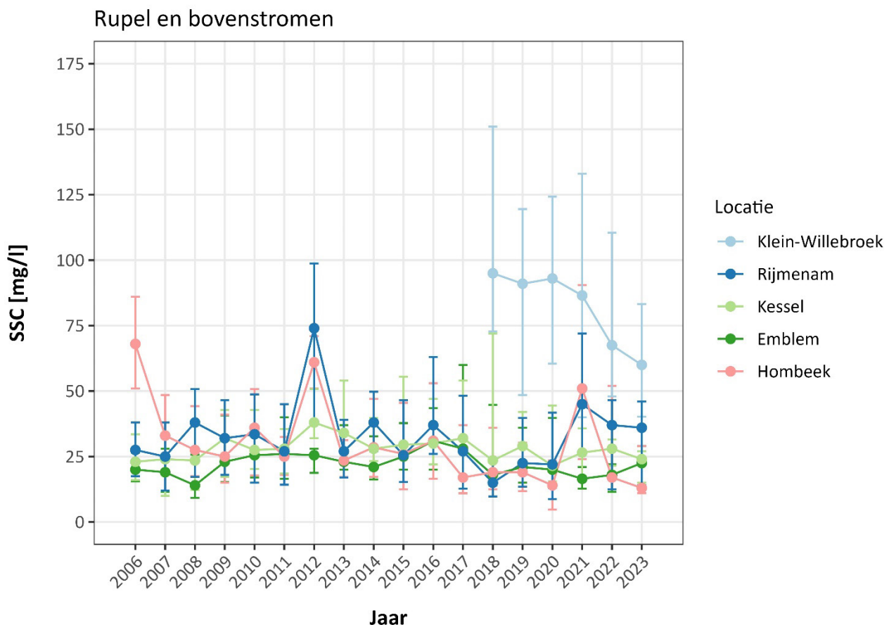
Figuur 62 – Evolutie jaarwaarden sedimentconcentratie nabij wateroppervlak (markers = mediaan, error bars = P25 en P75) voor de meetlocaties in de Rupel en randen tijgebied in het Rupelbekken.
