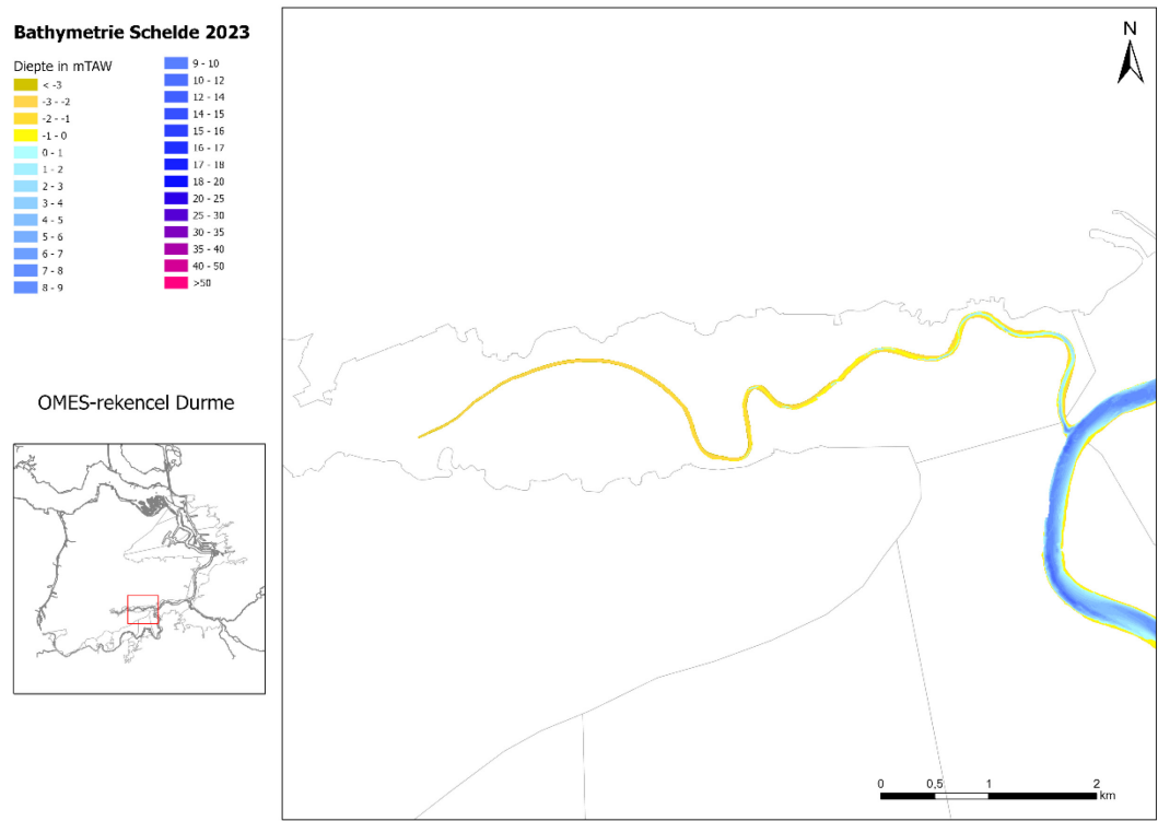
Figuur 117 – Topo-bathymetrie 2023 OMES-segment Durme.
