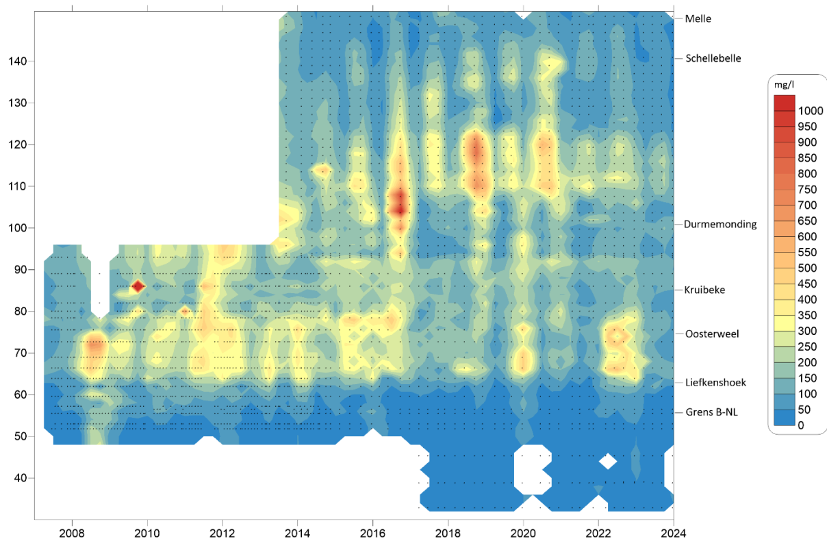
Figuur 66 – Sedimentconcentratie nabij het oppervlak (mg/l) bij halftij-eb langs de Zeeschelde (interpolatietechniek: Kriging, zoekradius X-as: 0,25 jaar, zoekradius Y-as: 2 km)
