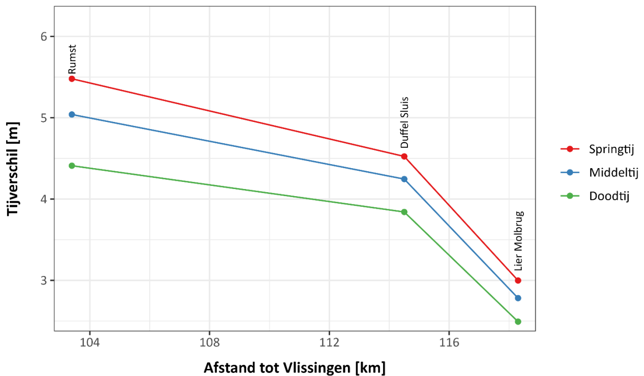
Figuur 6 – Gemiddeld tijverschil (GTV) bij middeltij, springtij en doottij in 2023 voor de Beneden-Nete.
