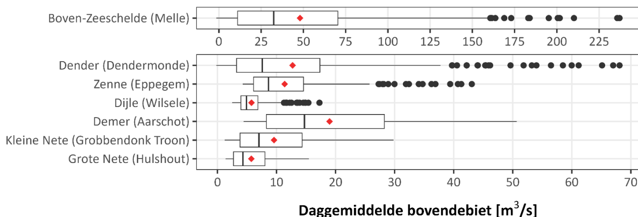
Figuur 19 – Jaarwaarden 2023 voor de stations aan de randen van het tijgebied. Rode ruit geeft de gemiddelde waarde aan. Individuele daggemiddelde bovendebiten die buiten het P10-P90 interval vallen, worden als zwarte punten weergegeven.
