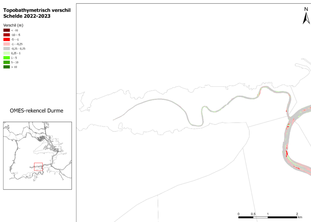
Figuur 127 – Verschilkaart 2022-2023 OMES-segment Durme.
