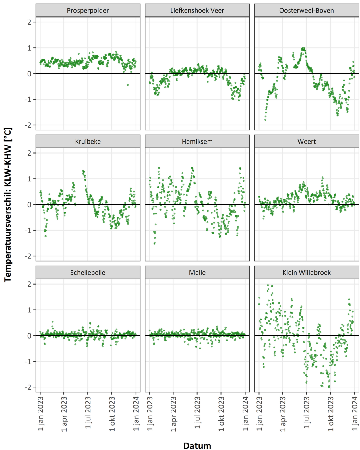
Figuur 42 – Seizoenaal verloop temperatuursverschil tussen KLW en KHW (gemiddeldes KLW min gemiddeldes KHW) voor de verschillende meetstations.
