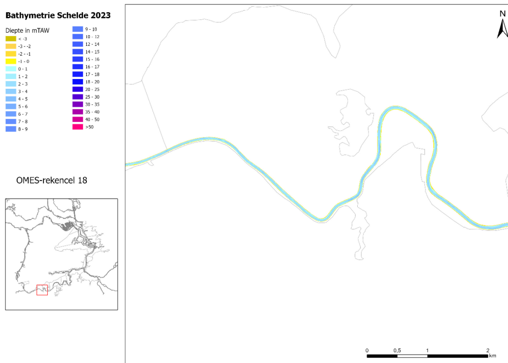
Figuur 115 – Topo-bathymetrie 2023 Zeeschelde: OMES-segment 18.
