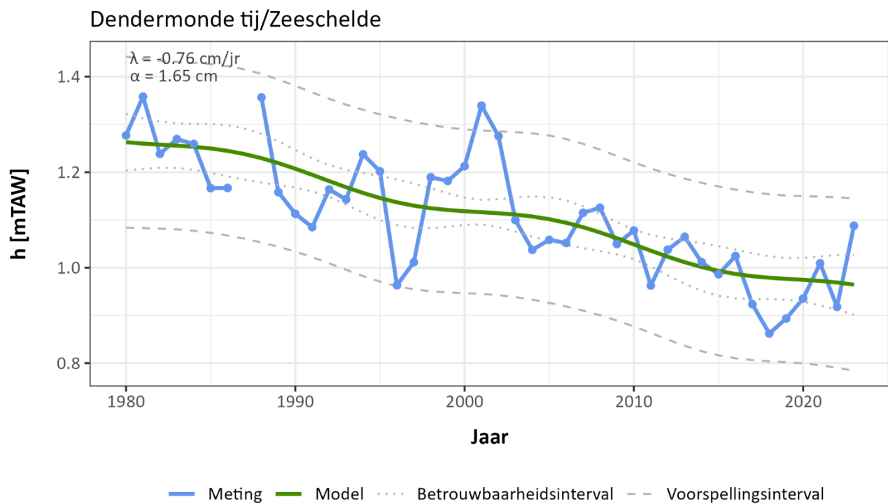
Figuur 98 –Trend jaargemiddeld laagwater te Dendermonde bepaald over de periode 1980-2023.
