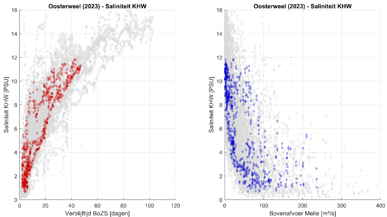
Figuur 48 – Relatie tussen de saliniteit te Oosterweel bij kentering hoogwater en de verblijftijd (links) en de bovenafvoer (rechts) Gekeurde markers tonen waarden voor het laatste jaar (2023), grijze markers is de periode hiervoor.
