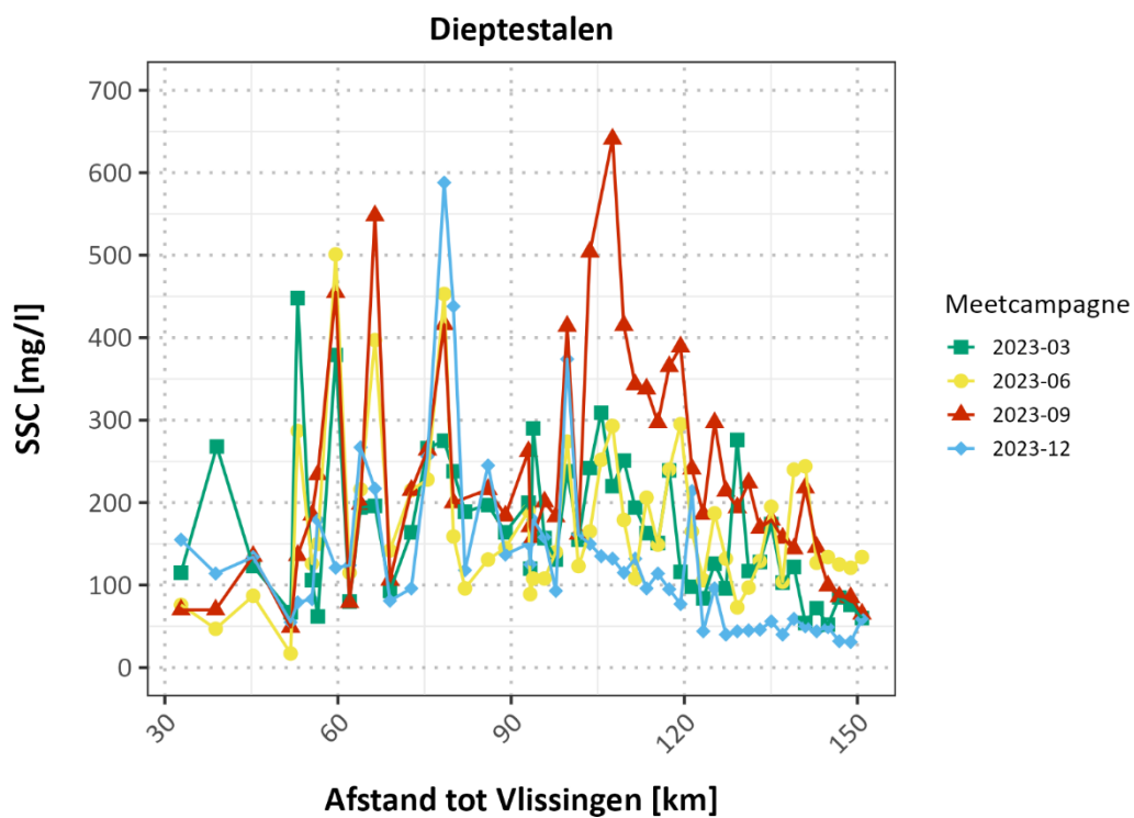
Figuur 65 – Sedimentconcentratie aan de bodem bij halftij-eb langsheen de volledige Zeeschelde
