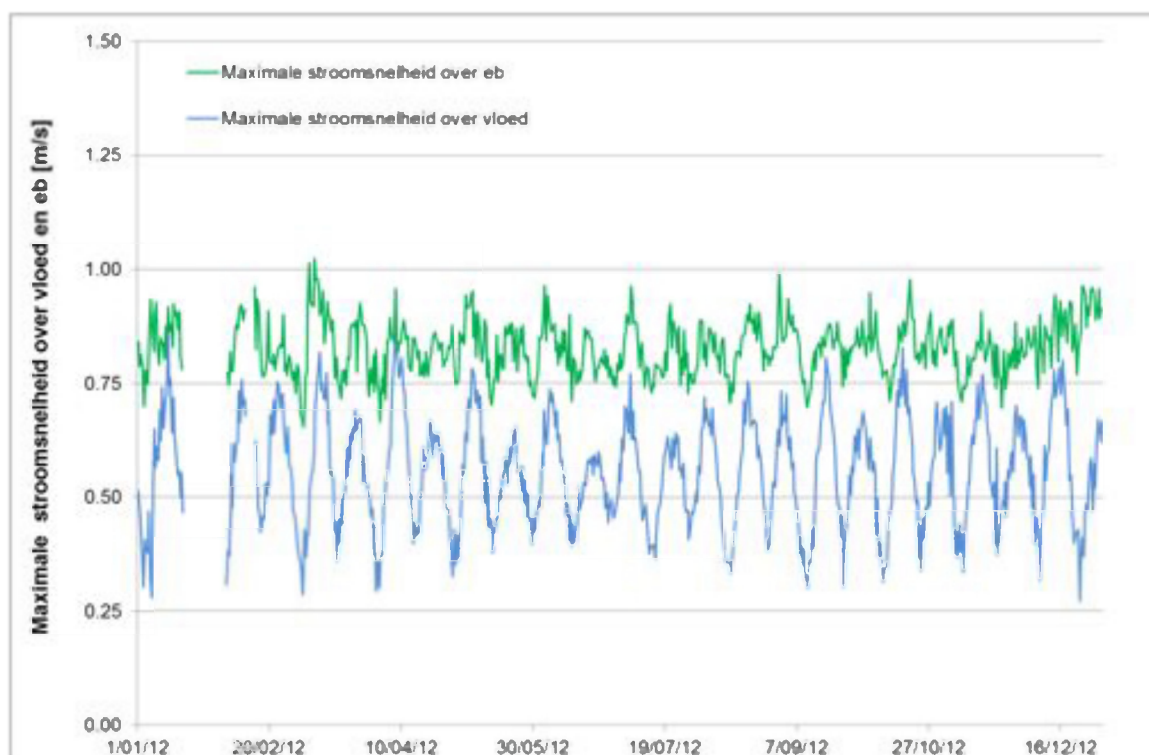
Figuur 64 - Maximale stroomsnelheid over vloed en over eb te Driegoten (Boven-Zeeschelde)
