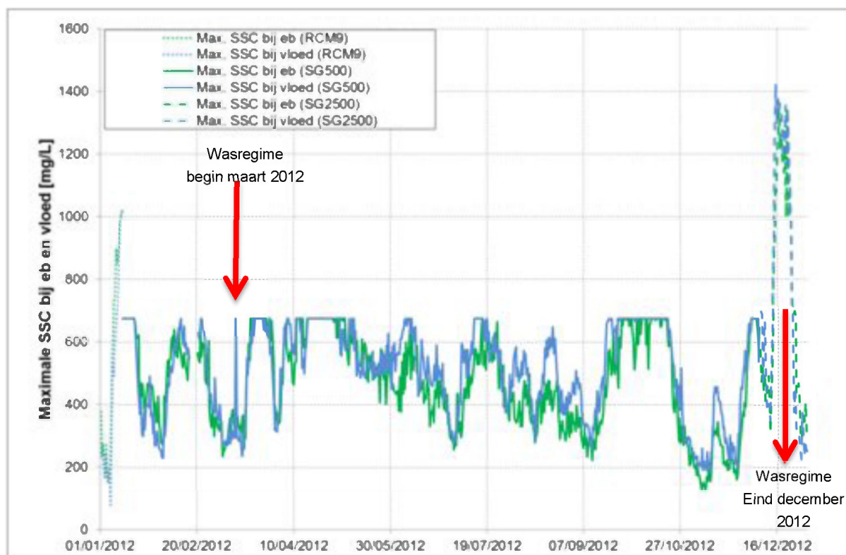
Figuur 118 - Maximale SSC bij eb en vloed te Oosterweel (Beneden-Zeeschelde), bovenste meettoestel
