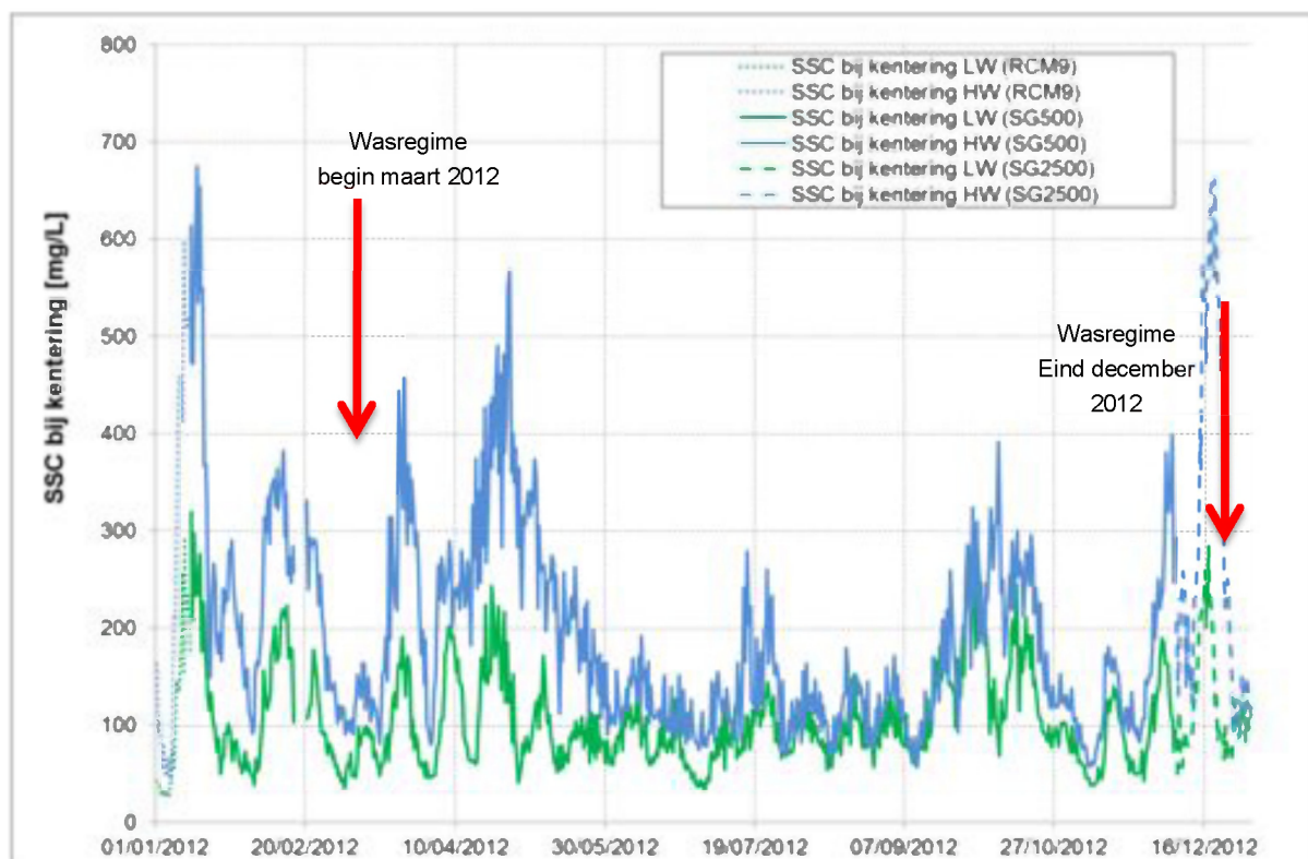
Figuur 111 - SSC bij KLW en KHW te Oosterweel (Beneden -Zeeschelde), bovenste meettoestel
