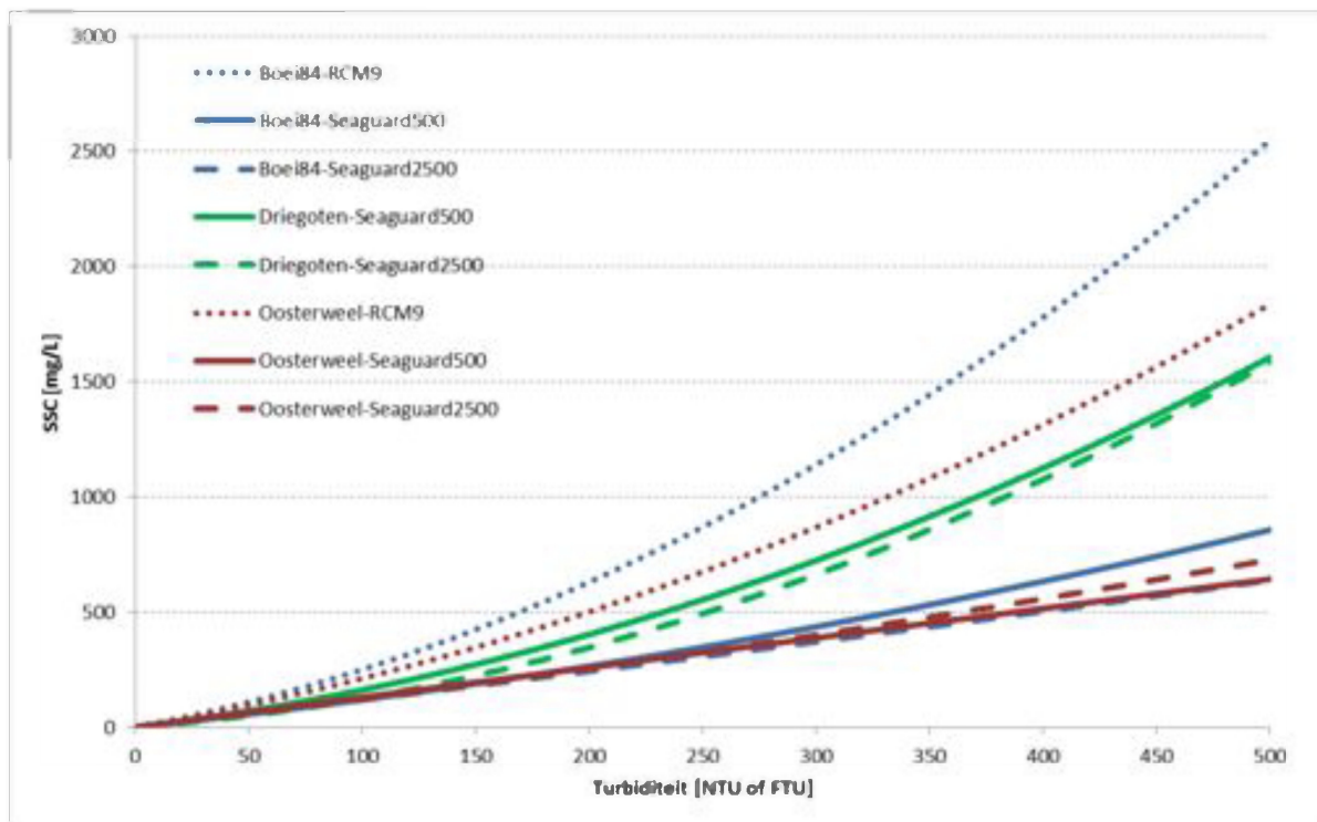
Figuur 108 - Kalibratiereferenties (Turbiditeit – SSC) opgesteld voor Aanderaa RCM9 en Seaguard toestellen ter hoogte van meetlocaties Boei 84, Oosterweel en Driegoten
