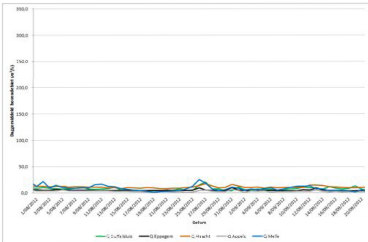
Figuur 46 - Zeescheldebekken: afvoer aan de meetraaien in de periode half april – half juli 2011
