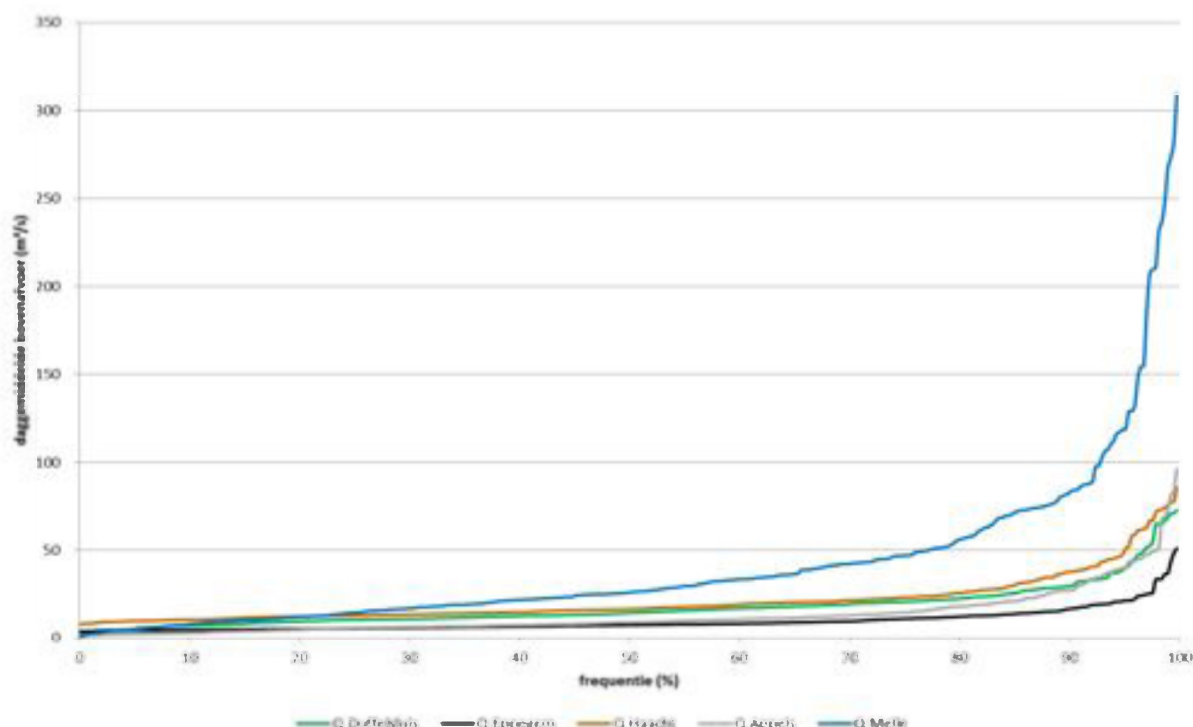
Figuur 35 - Zeescheldebekken: sortering naar grootte van de daggemiddelde bovendebielen aan de meetraaien, over het ganse jaar 2012
