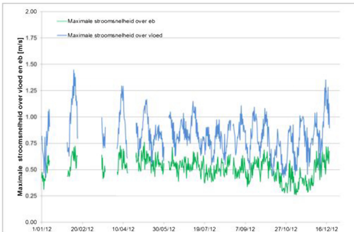
Figuur 61 - Maximale stroomsnelheid over vloed en over eb te Boei84 (Beneden-Zeeschelde), onderste meettoestel
