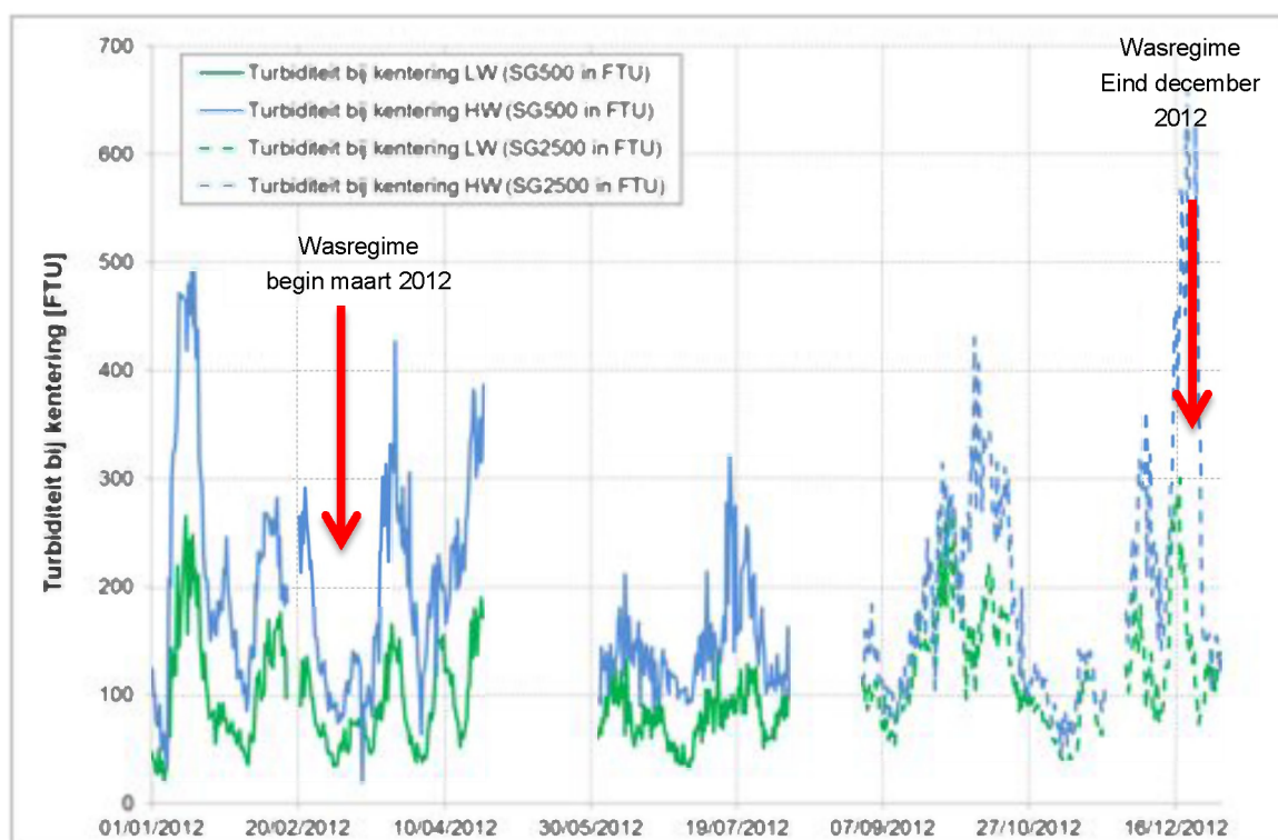
Figuur 94 - Turbiditeit bij KHW en KLW te Oosterweel (Beneden-Zeeschelde), onderste meettoestel
