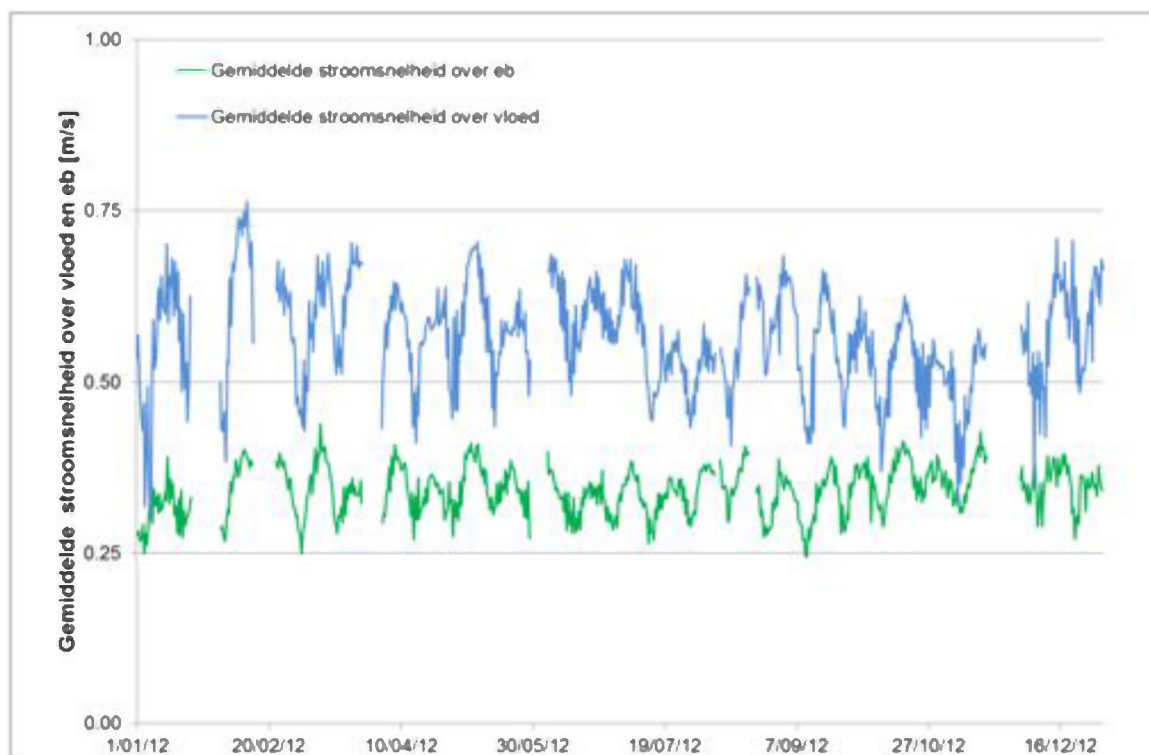
Figuur 55 - Gemiddelde stroomsnelheid over vloed en over eb te Boei 84 (Beneden-Zeeschelde), bovenste meettoestel
