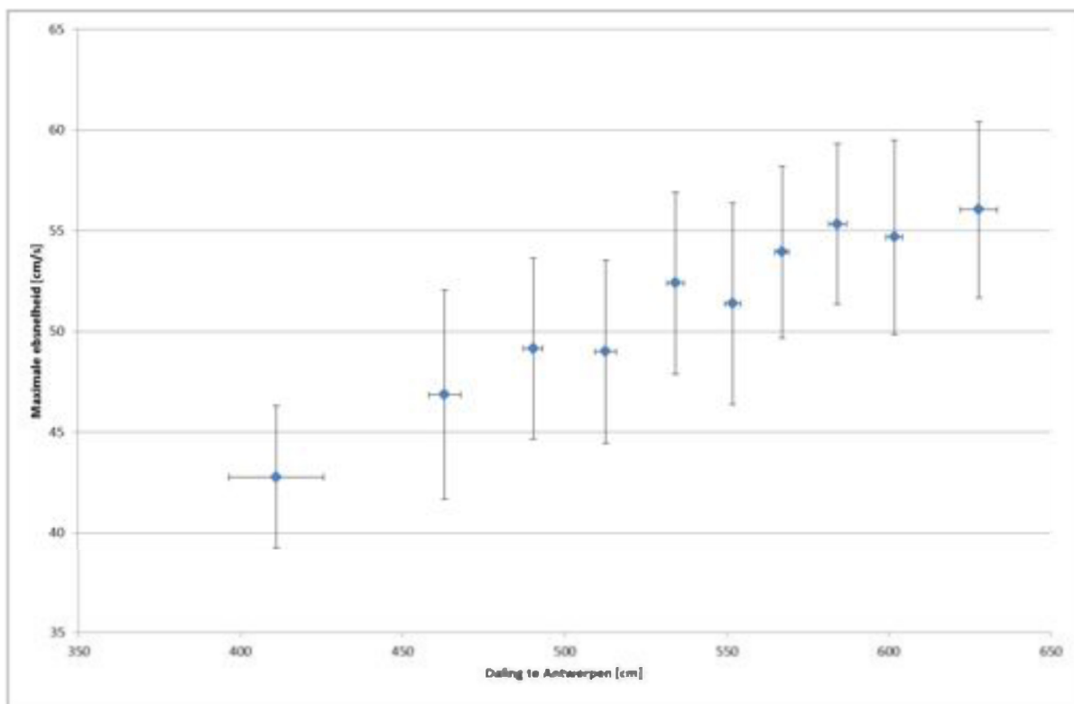
Figuur 68 - Maximale ebsnelheid te Boei 84 (Beneden-Zeeschelde), onderste meettoestel, versus de daling in waterpeil te Antwerpen
