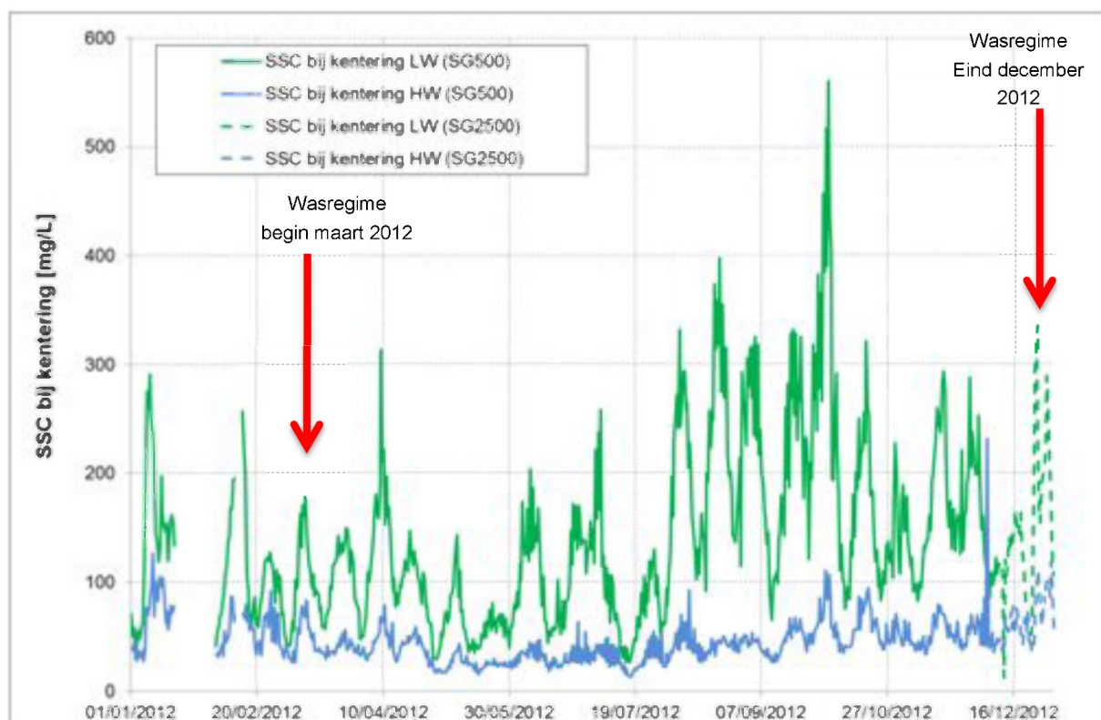
Figuur 113 - SSC bij K LW en K HW te Driegoten (Boven-Zeescheldebekken)
