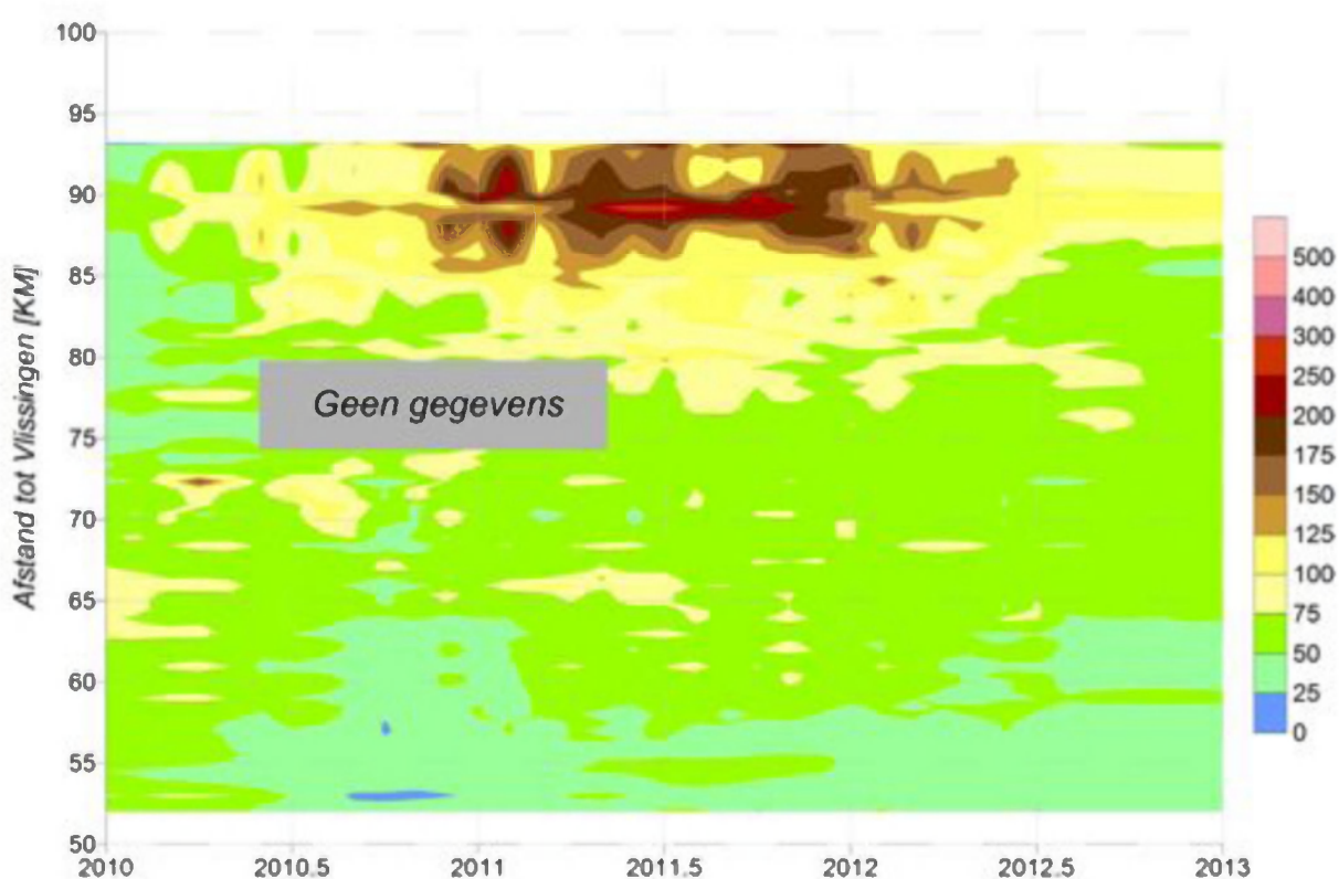
Figuur 136 - Sedimentconcentratie bij kentering hoogwater langsheen de Beneden Zeeschelde
