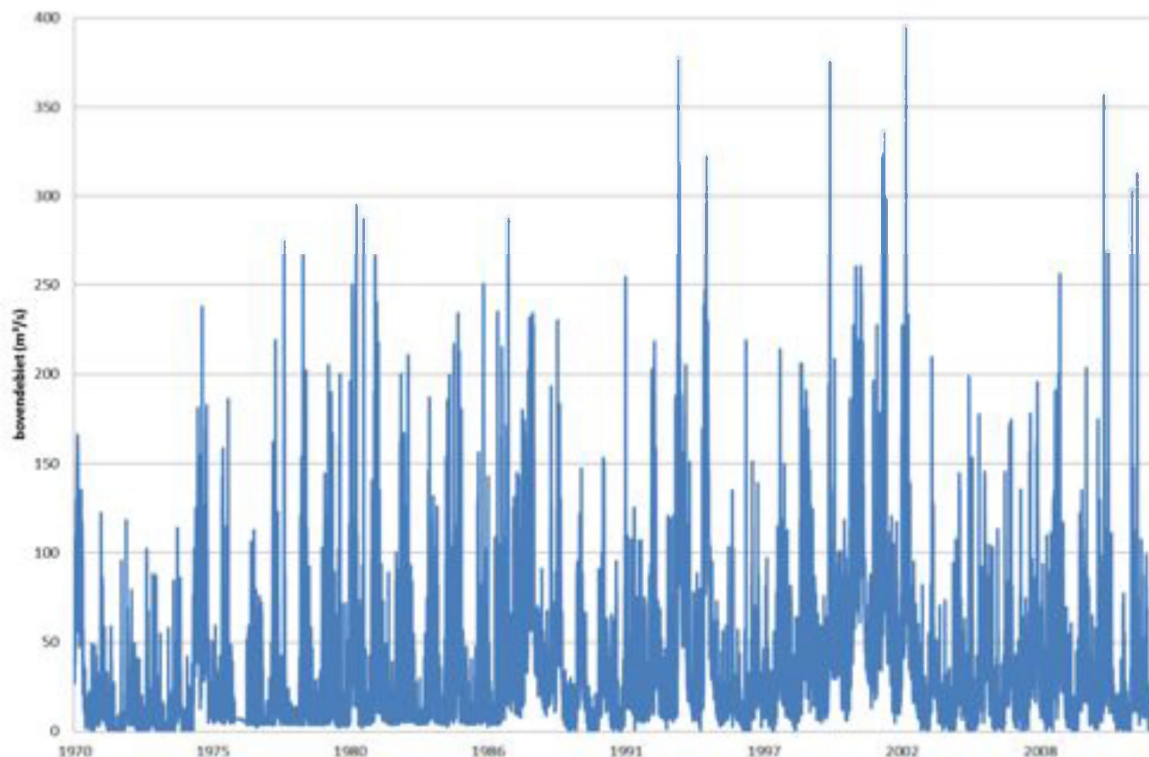
Figuur 47 - Zeescheldebekken: verloop van de daggemiddelde bovendebieten in de Zeeschelde te Melle periode 1970-2011 (alle bovendebieten in m³/s)
