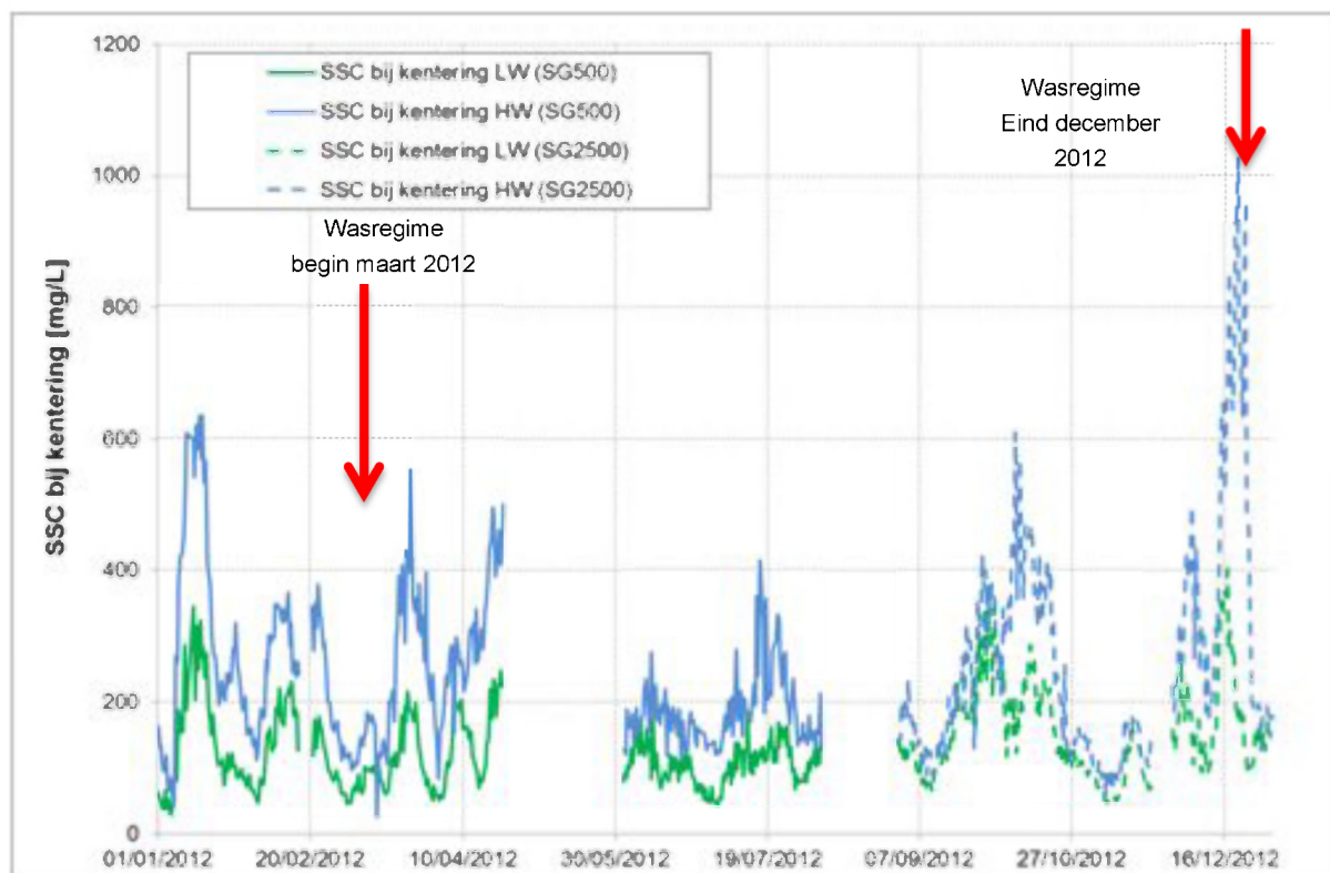
Figuur 112 - SSC bij K LW en K HW te Oosterweel (Beneden-Zeescheldebekken), onderste meettoestel
