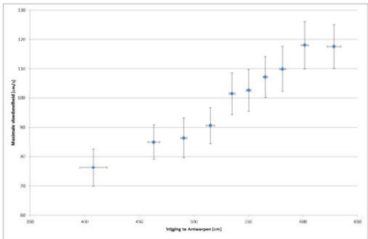
Figuur 67 - Maximale vloodsnelheid te Boei 84 (Beneden-Zeeschelde), bovenste meettoestel, versus de stijging in waterpeil te Antwerpen
