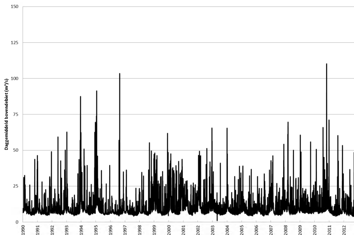
Figuur 51 - Zenne te Eppegem: verloop daggemiddelde afvoer over de periode 1990-2012
