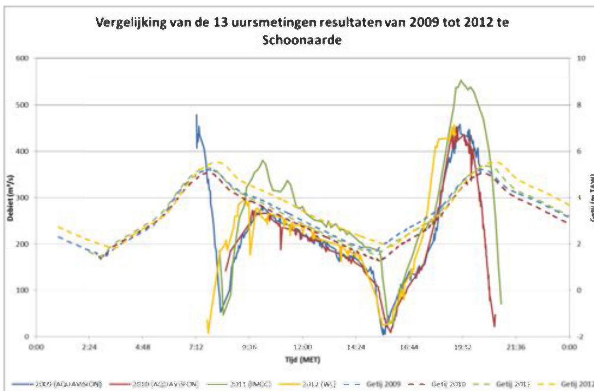
Figuur 163 - Debiet en getij tijdens de dertienuursmetingen te Schoonaarde (Boven-Zeeschelde) in 2009 t.e.m. 2012
