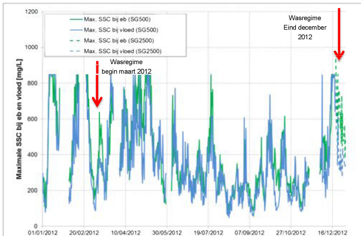
Figuur 114 - Maximale SSC bij eb en vloed te Boei 84 (Beneden-Zeescheldebekken), bovenste meettoestel
