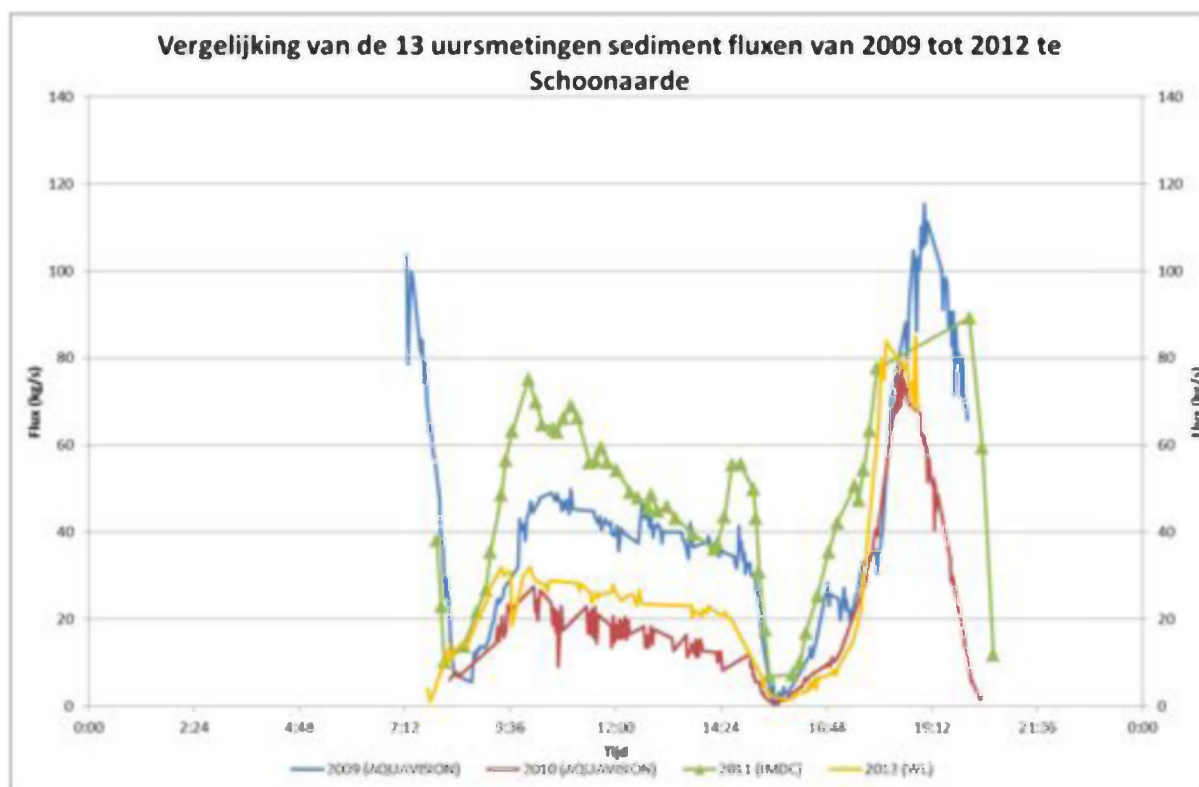
Figuur 165 - SSF tijdens de dertienuursmetingen te Schoonaarde (Boven-Zeeschelde) in 2009 t.e.m. 2012
