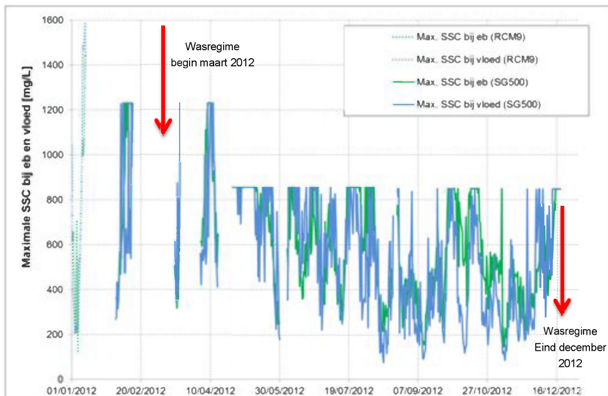
Figuur 115 - Maximale SSC bij eb en vloed te Boei 84 (Beneden-Zeescheldebekken), onderste meettoestel
