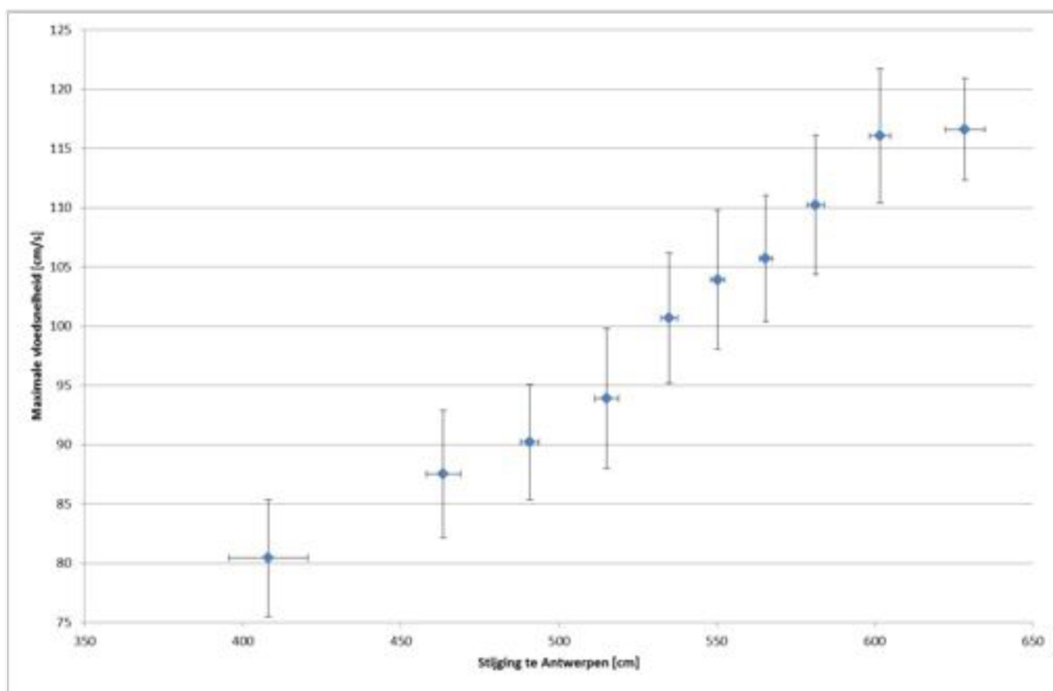
Figuur 71 - Maximale vloednelheid te Oosterweel (Beneden-Zeeschelde), bovenste meettoestel, versus de stijging in waterpeil te Antwerpen
