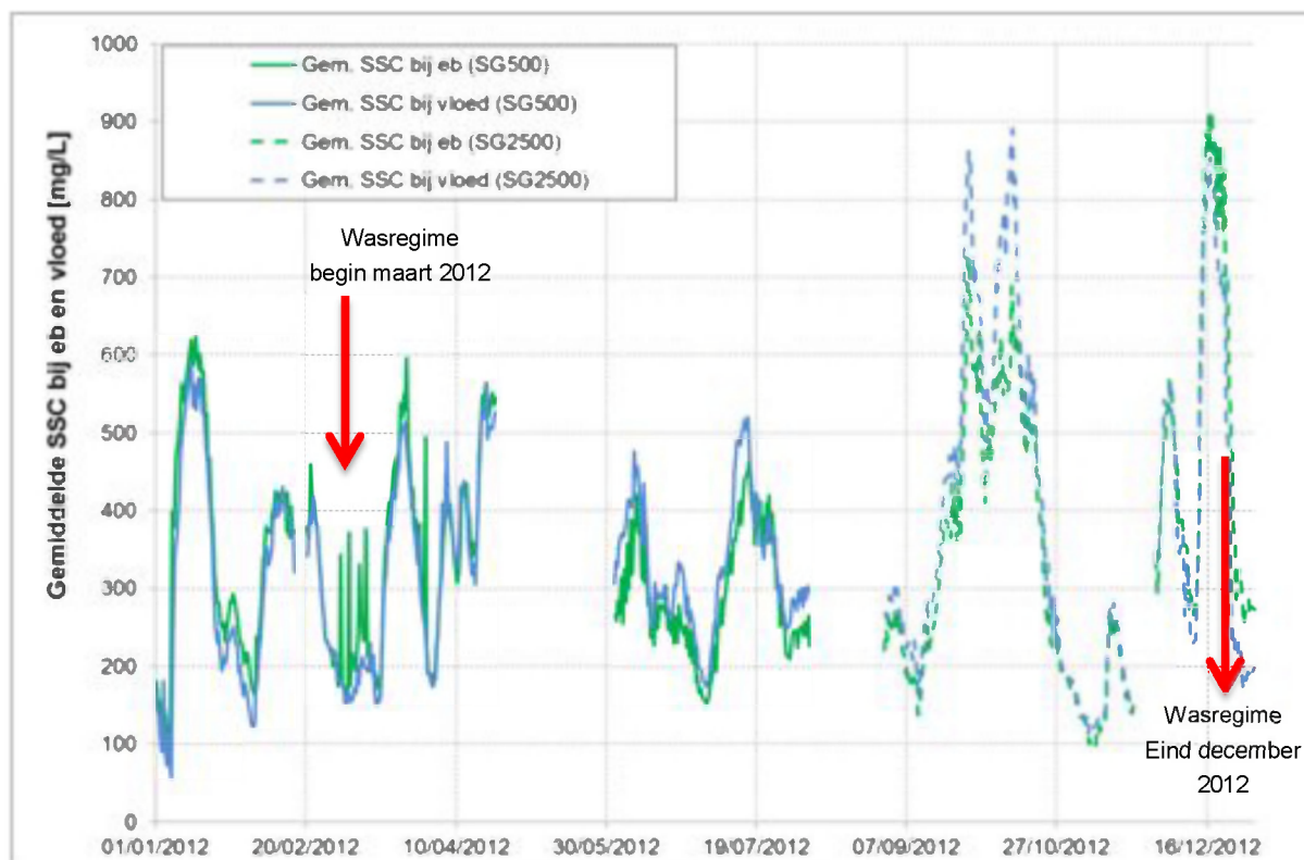
Figuur 121 - Gemiddelde SSC bij eb en vloed te Oosterweel (Beneden-Zeeschelde), onderste meettoestel
