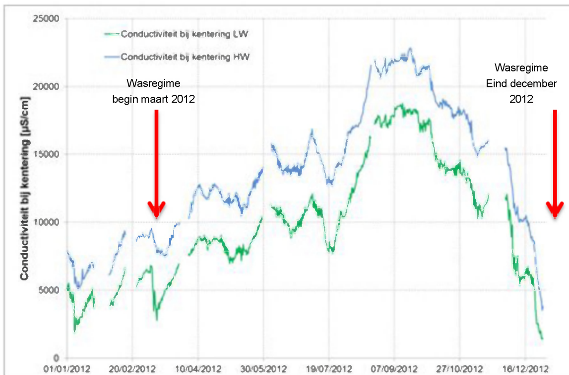
Figuur 83 - Conductiviteit bij KHW en KLW te Boei84 (Beneden- Zeeschelde), bovenste meettoestel
