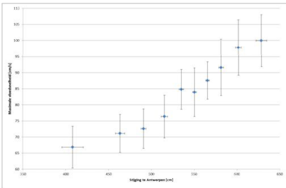
Figuur 69 - Maximale vloodsnelheid te Boei 84 (Beneden-Zeeschelde), onderste meettoestel, versus de stijging in waterpeil te Antwerpen
