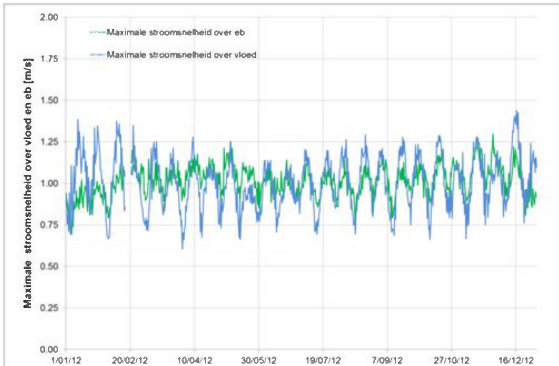
Figuur 62 - Maximale stroomsnelheid over vloed en over eb te Oosterweel (Beneden-Zeeschelde), bovenste meettoestel
