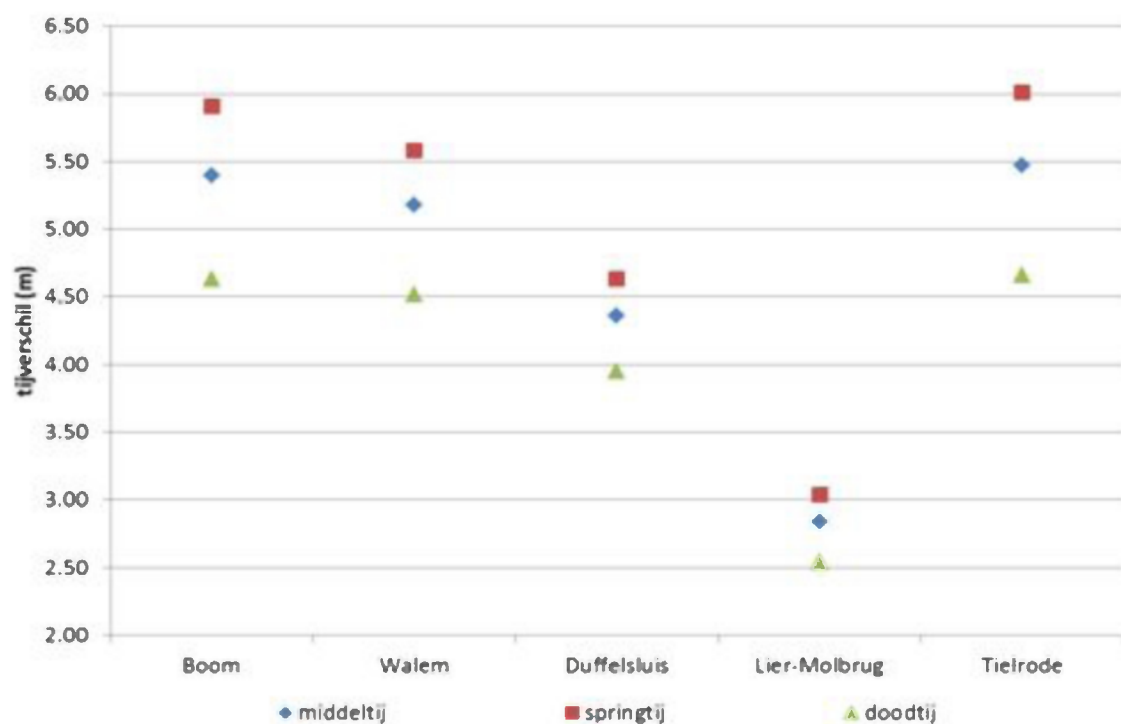
Figuur 14 - Gemiddeld tijvershil (GTV) bij middeltij, springtij en doodtij in 2012 voor de Rupel (Boom en Walem), Beneden Nete (Walem en Duffelsluis) en de Durme (Tielrode)
