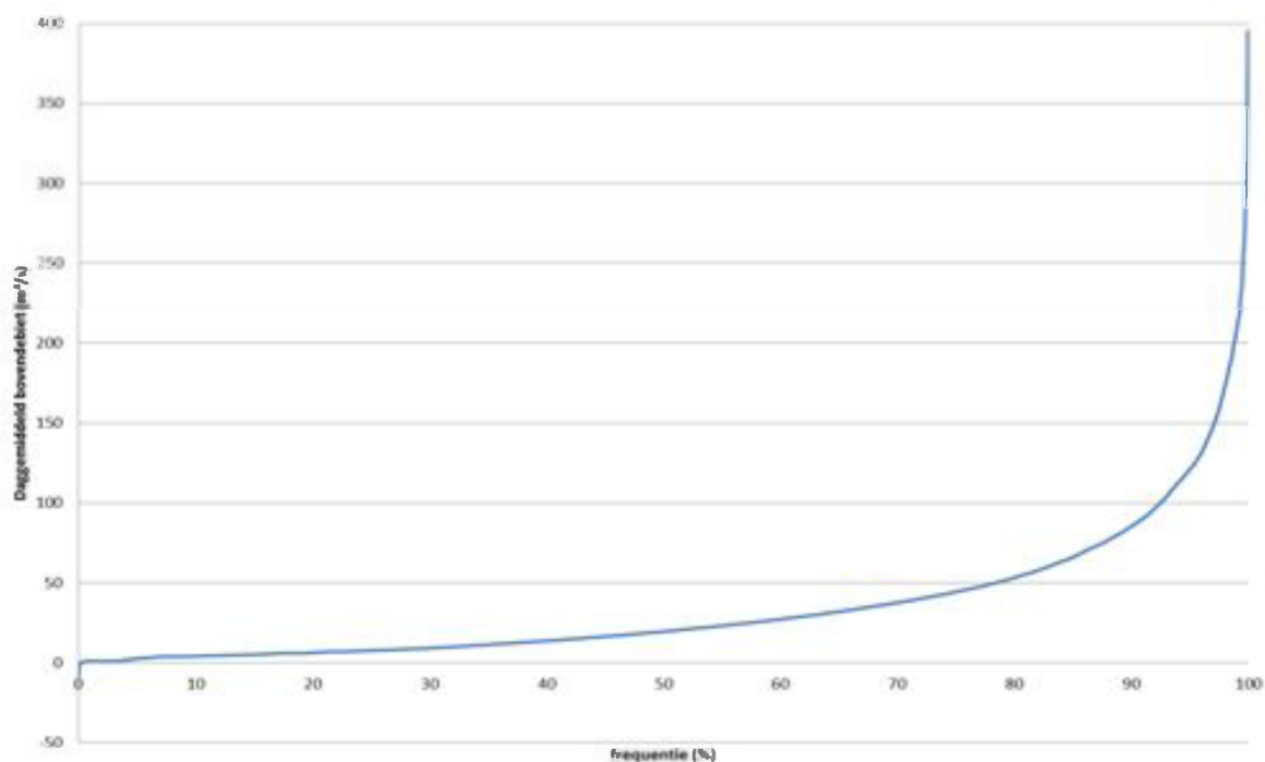
Figuur 48 - Zeescheldebekken: in grootte gerangschikt verloop van de daggemiddelde bovendebielen in de Zeeschelde te Melle over de periode 1970-2012 (alle bovendebielen in m³/s)
