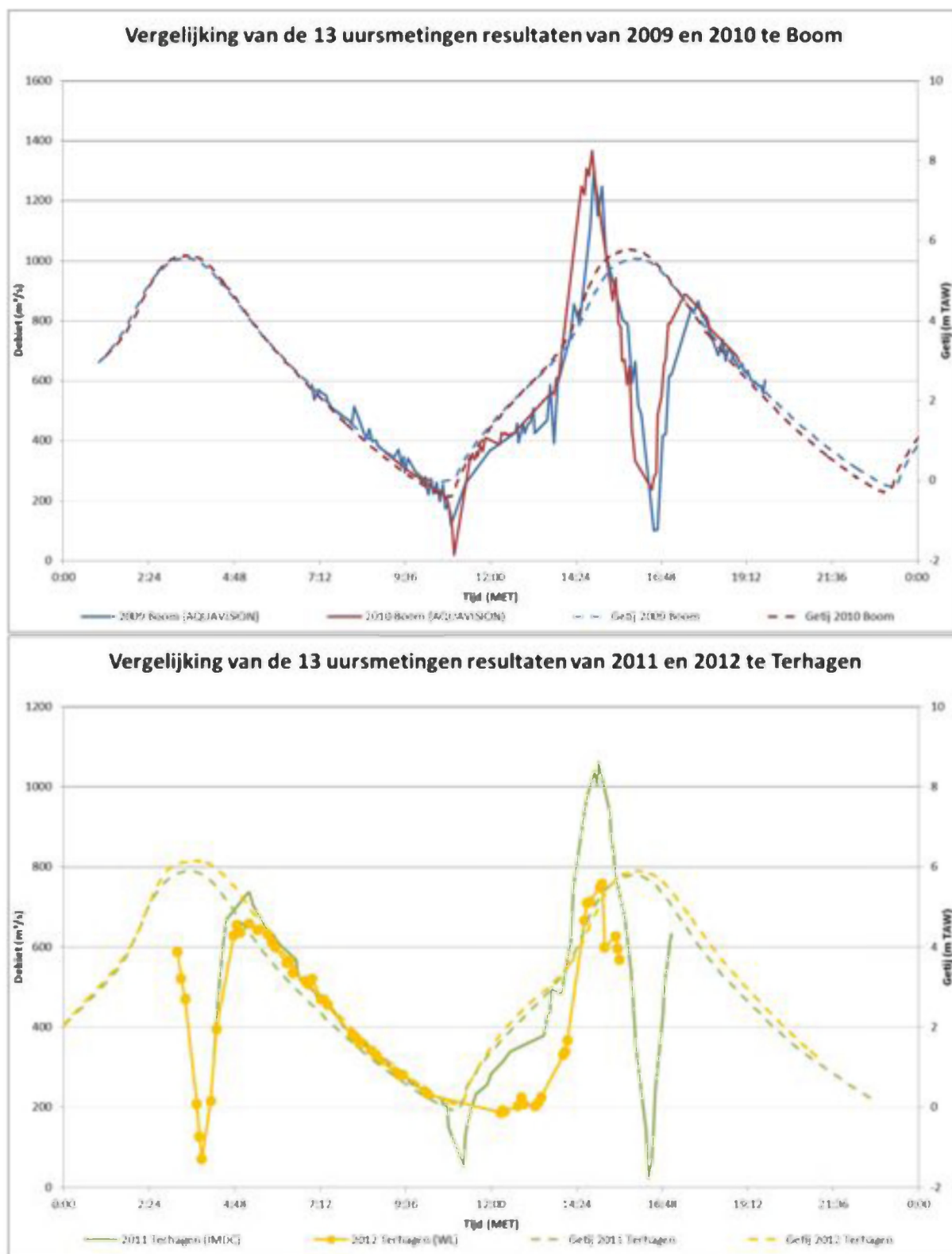
Figuur 167 - Debiet en getij tijdens de dertienuursmetingen te Boom en Terhagen (Rupel) in 2009 t.e.m. 2012
