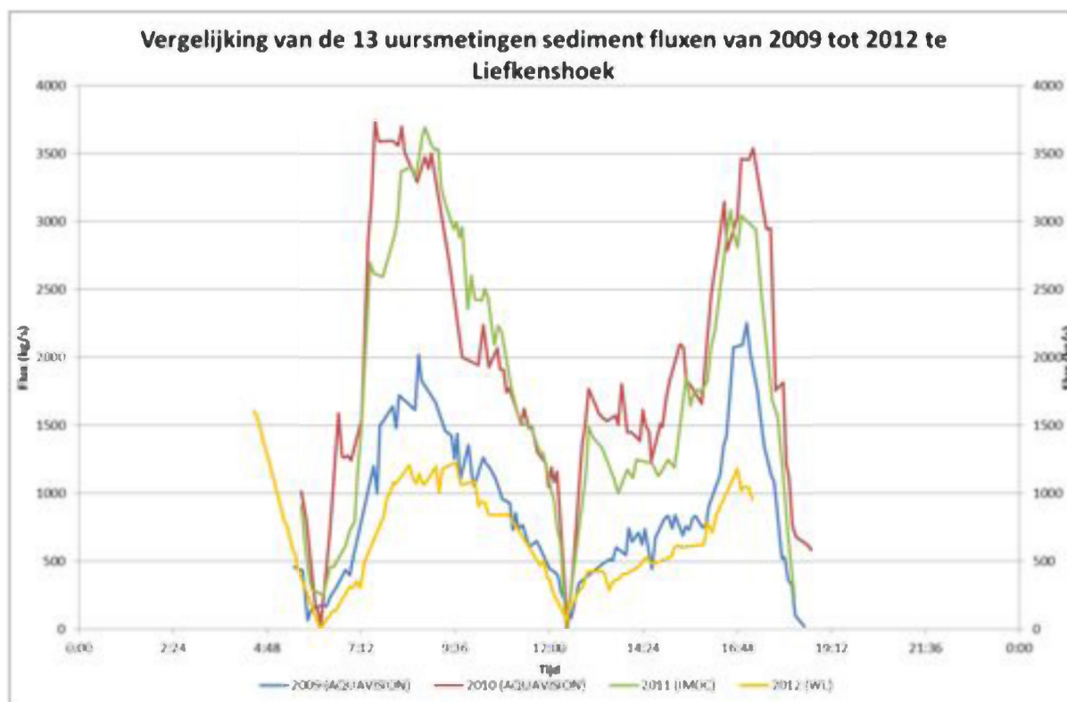
Figuur 148 - SSF tijdens de dertienuursmetingen te Liefkenshoek (Beneden-Zeeschelde) in 2009 t.e.m. 2012
