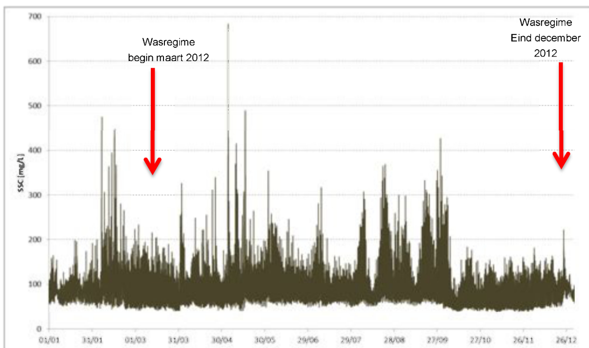
Figuur 132 - SSC (berekend uit turbiditeit) te Duffelsluis (Beneden-Nete)
