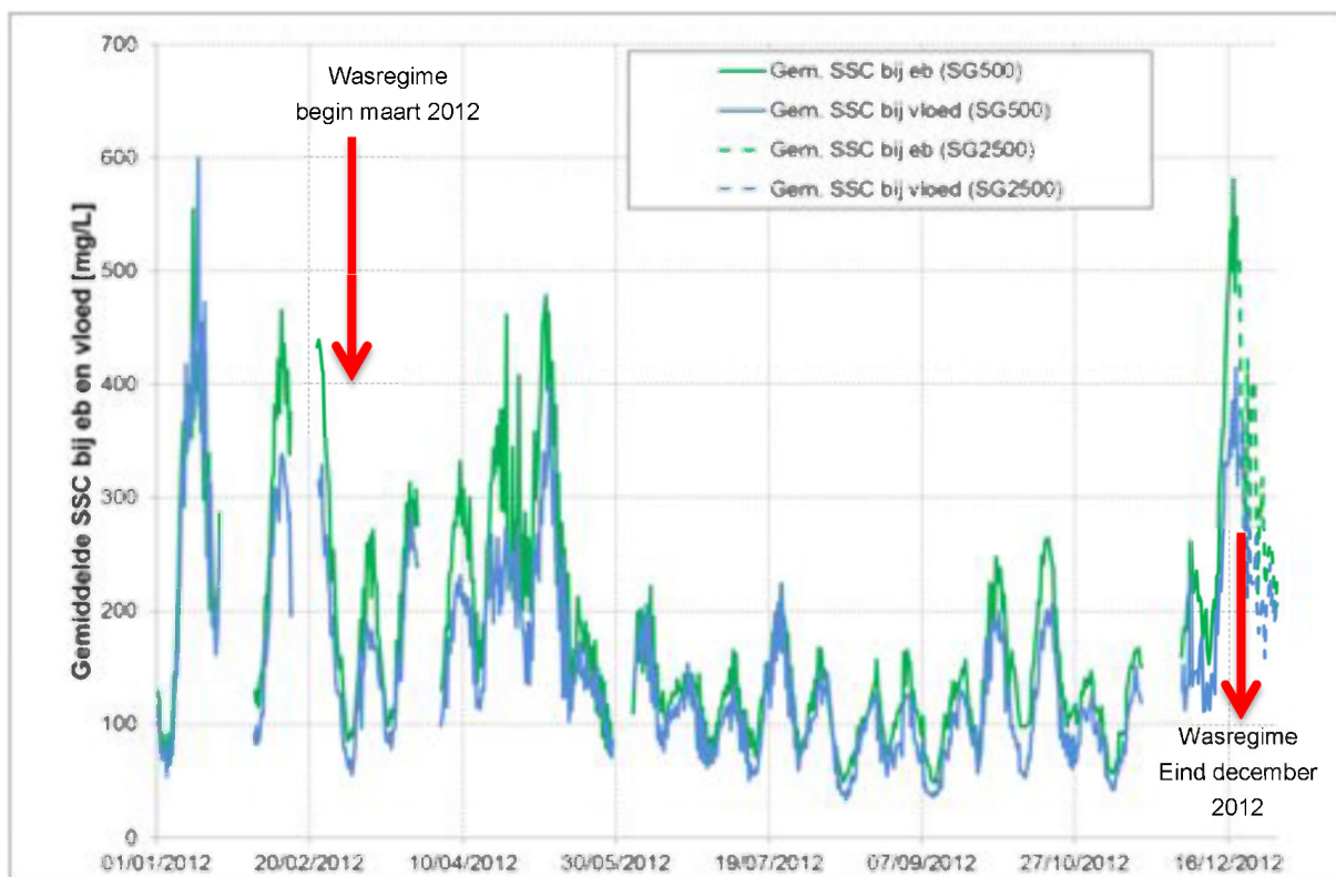
Figuur 116 - Gemiddelde SSC bij eb en vloed te Boei 84 (Beneden-Zeeschelde), bovenste meettoestel
