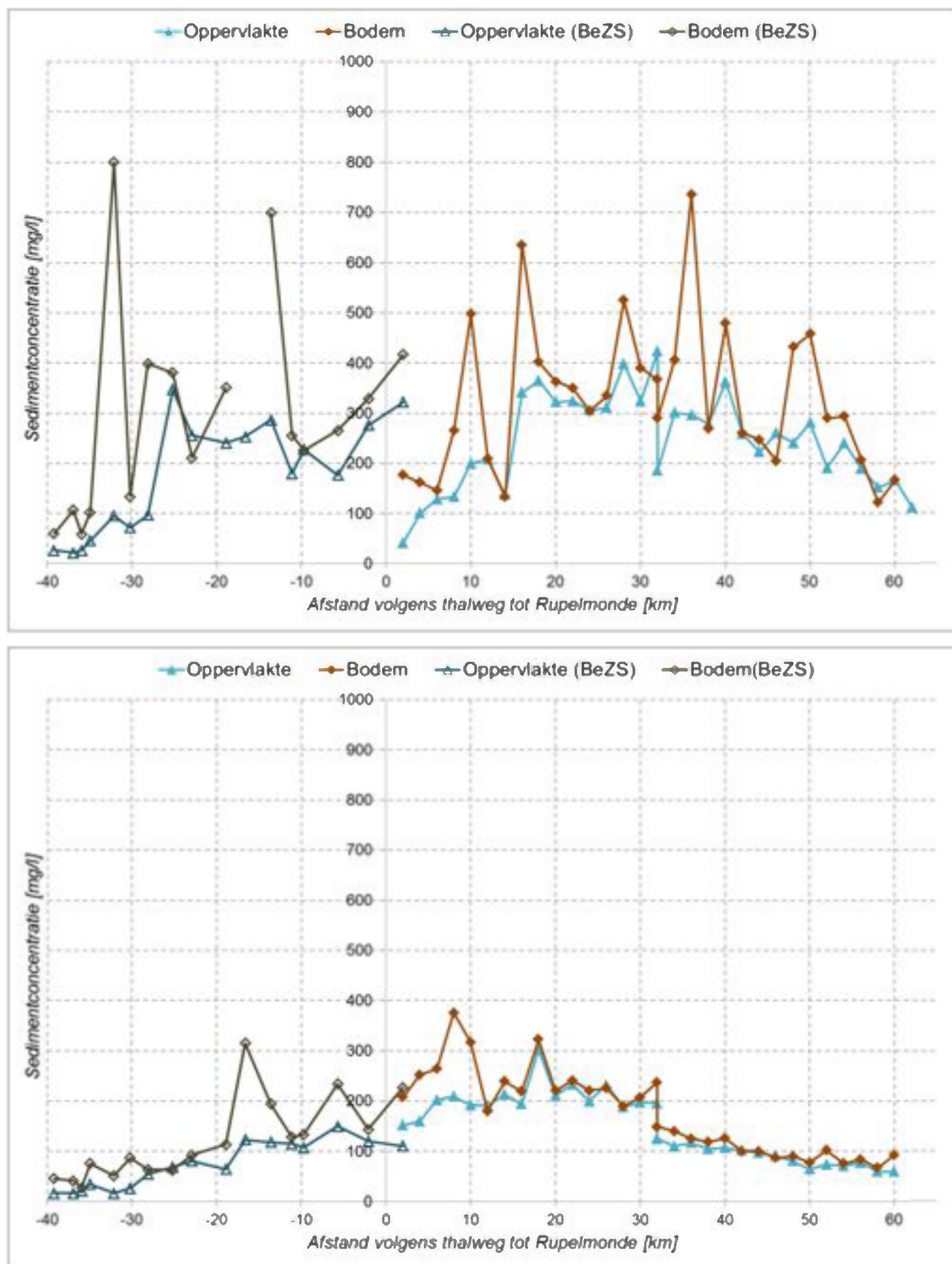
Figuur 139 - Sedimentconcentratie bij half-tij-eb langsheen de volledige Zeeschelde Boven: 08/2012 | onder 11/2012 (uit Plancke et al. , 2013)
