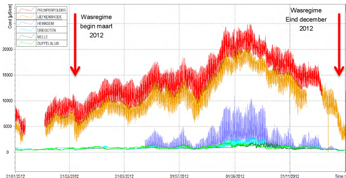
Figuur 90 - Conductiviteit bij heersende temperatuur te Prosperpolder en Liefkenshoek (Beneden-Zeeschelde), Hemiksem, Driegoten en Melle (Boven-Zeeschelde) en Duffelsluis (Beneden-Nete)
