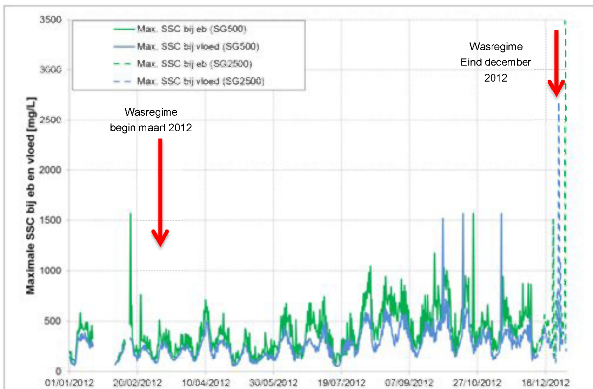
Figuur 122 - Maximale SSC bij eb en vloed te Driegoten (Boven-Zeeschelde)
