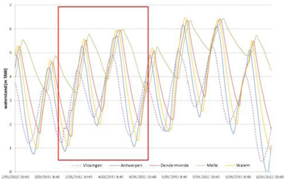
Figuur 18 - Tij te Antwerpen, Dendermonde, Melle, Walem en Vlissingen: tijverloop van 2 t.e.m. 6 januari 2012
