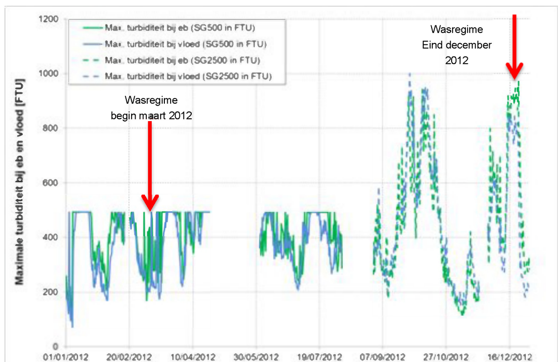
Figuur 101 - Maximale turbiditeit bij eb en vloed te Oosterweel (Beneden-Zeeschelde), onderste meettoestel
