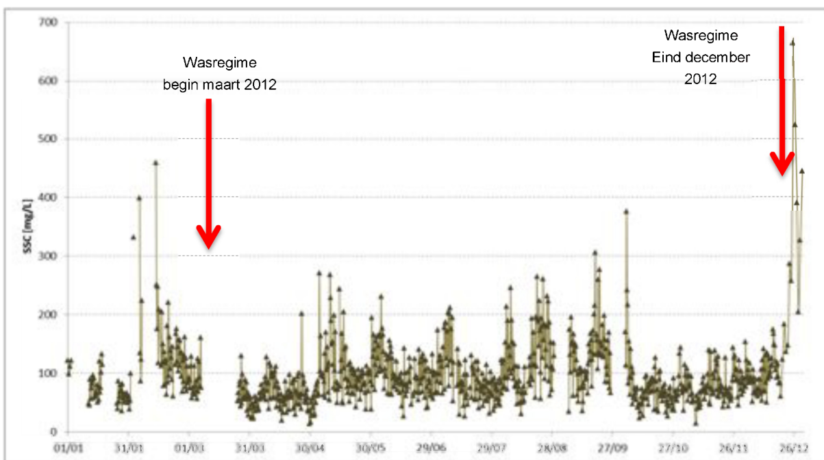
Figuur 128 - SSC (gemeten m.b.v. automatische staalname) te Duffelsluis (Beneden-Nete)
