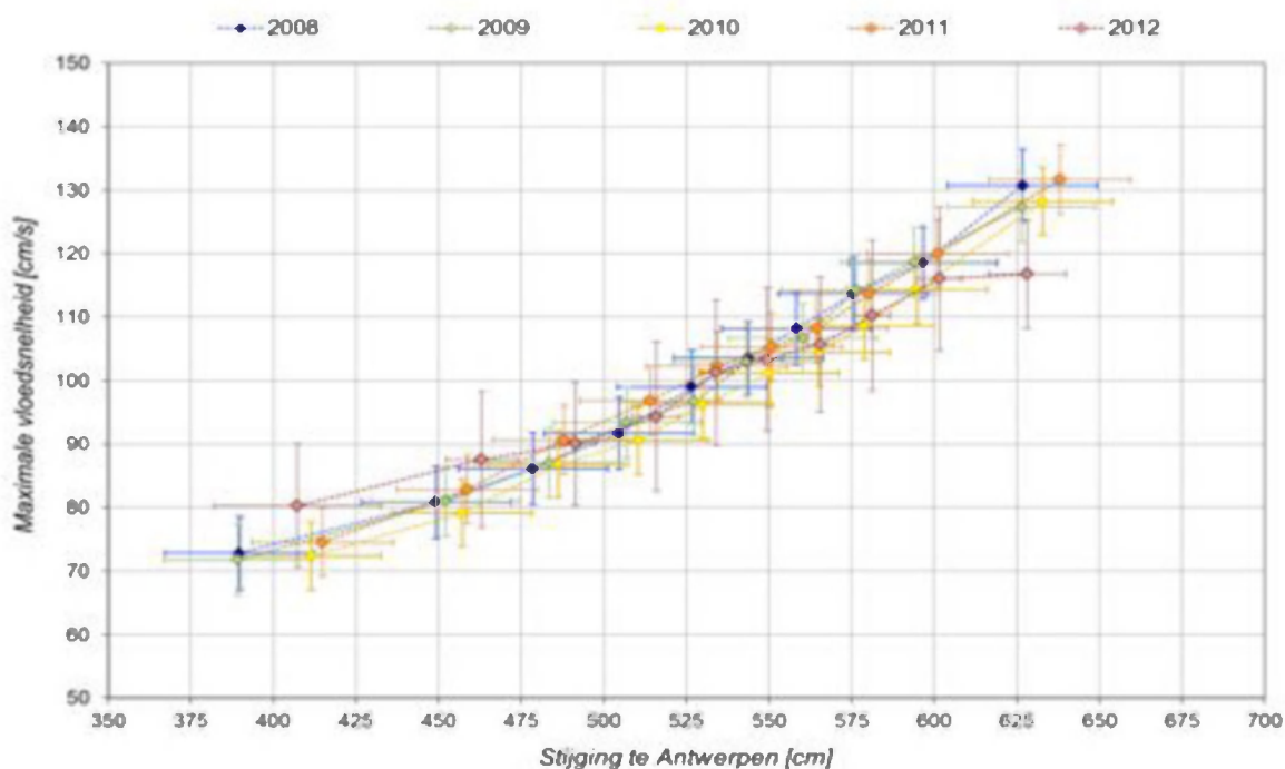
Figuur C2- 2: Maximale vloodsnelheid te Oosterweel (Beneden-Zeeschelde), bovenste meettoestel, versus de stijging in waterpeil te Antwerpen
