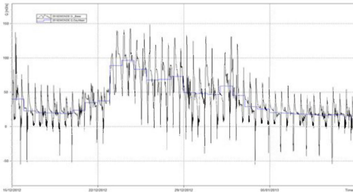
Figuur 44 - Evolutie van de continue (5-minuutgemiddelde) en daggemiddelde debieten op de Dender te Dendermonde voor de periode 15/12/2012 – 11/01/2013
