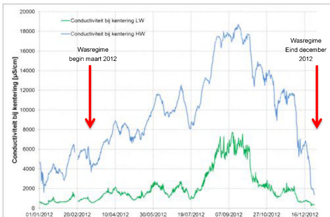
Figuur 85 - Conductiviteit bij KHW en KWL te Oosterweel (Beneden- Zeeschelde), bovenste meettoestel
