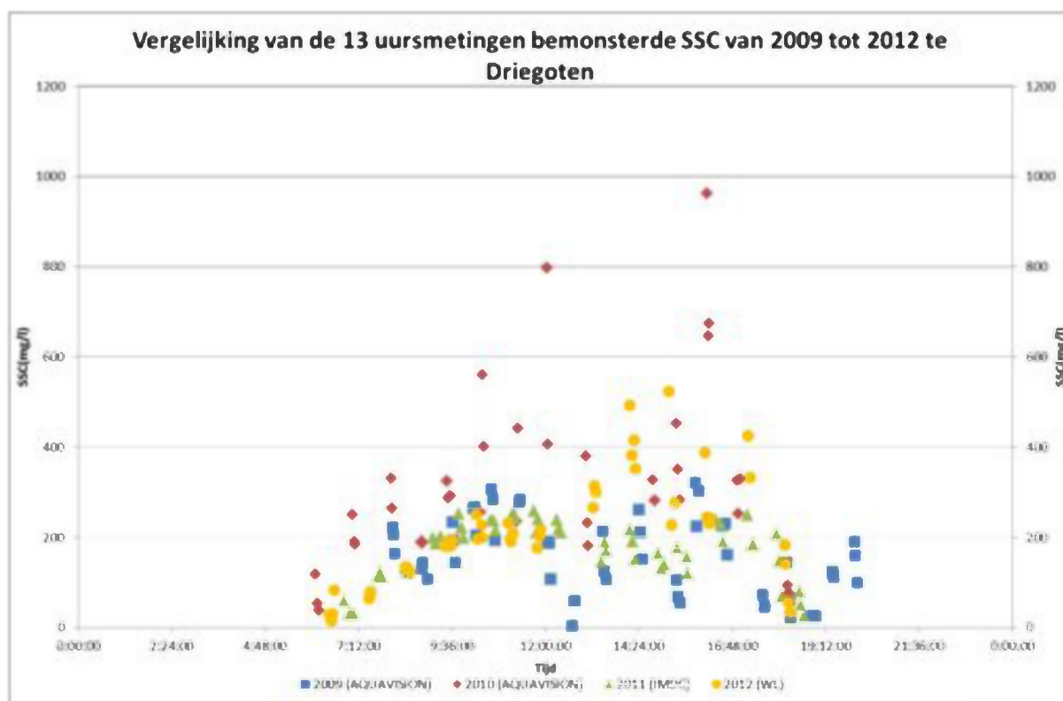
Figuur 160 - Gemeten SSC tijdens de dertienuursmetingen te Driegoten (Boven-Zeeschelde) in 2009 t.e.m. 2012
