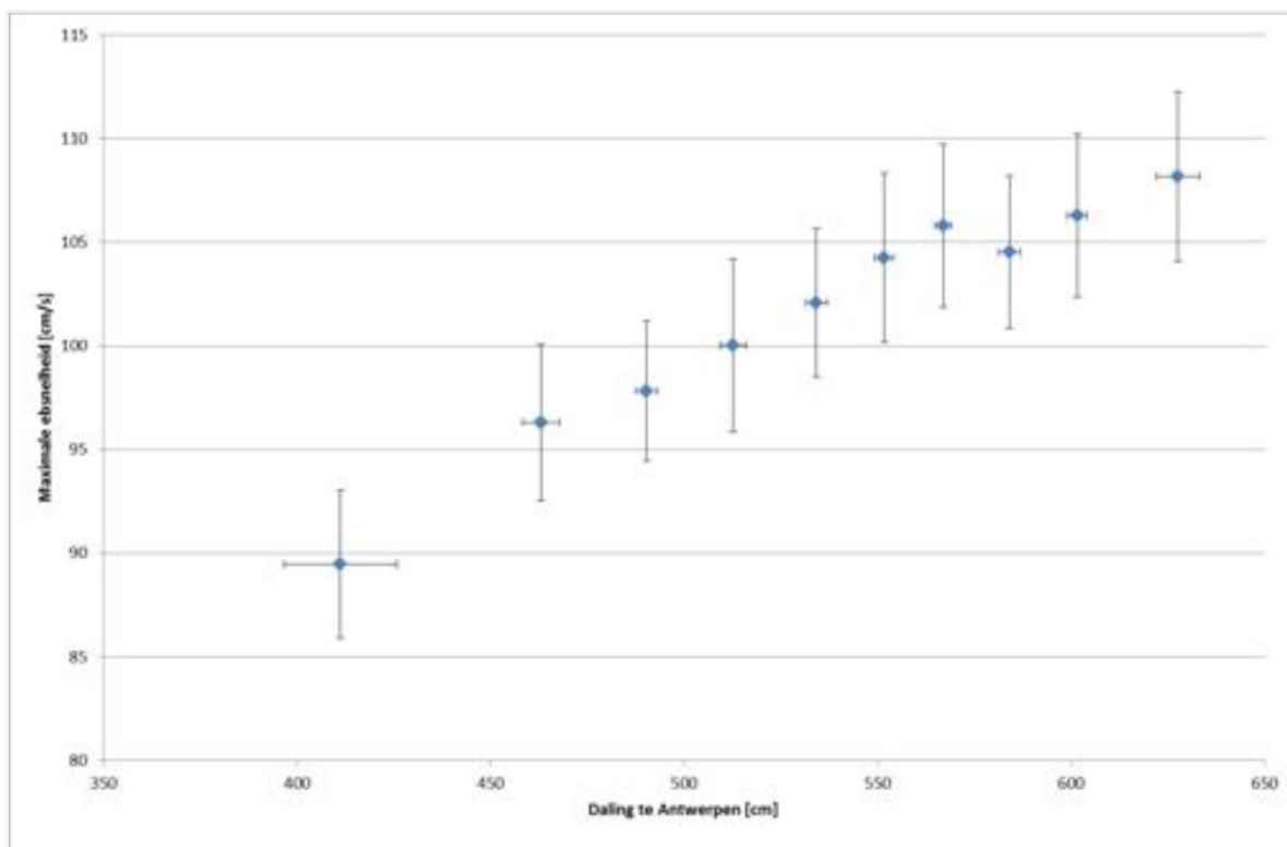
Figuur 70 - Maximale ebsnelheid te Oosterweel (Beneden-Zeeschelde), bovenste meettoestel, versus de daling in waterpeil te Antwerpen
