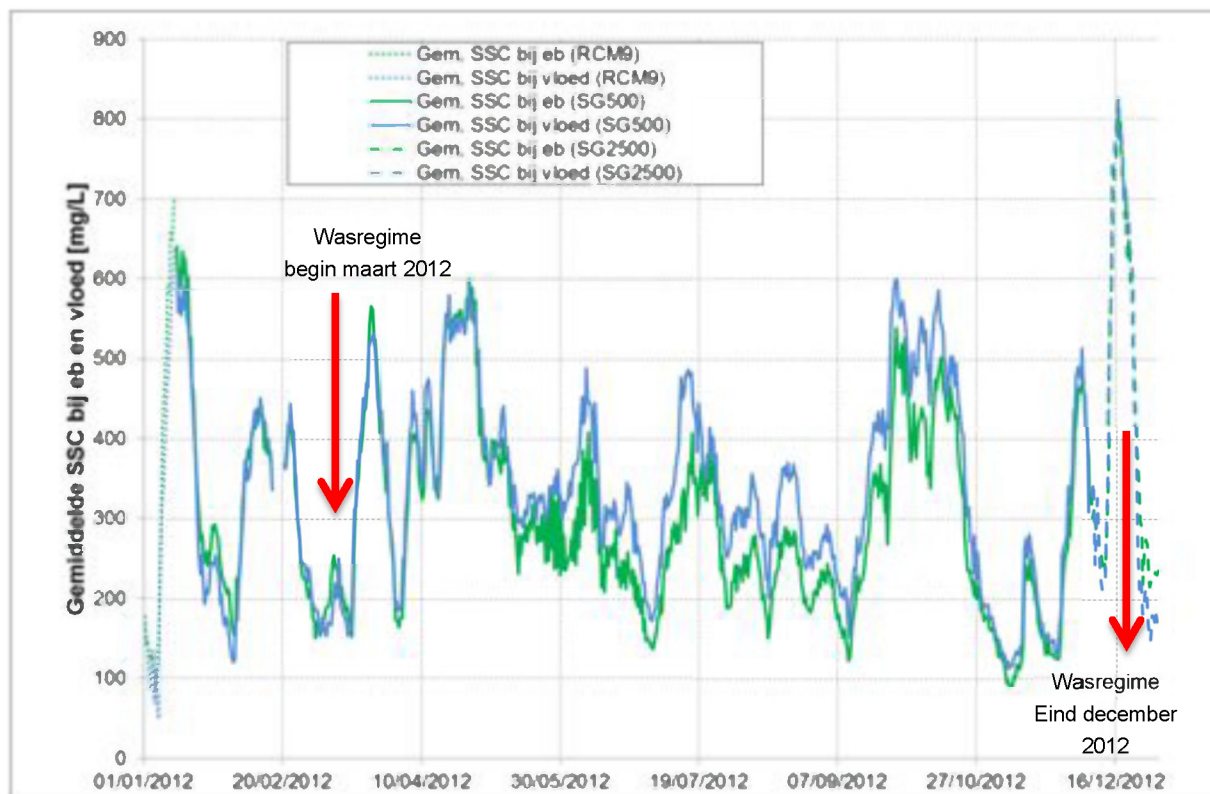
Figuur 120 - Gemiddelde SSC bij eb en vloed te Oosterweel (Beneden-Zeeschelde), bovenste meettoestel
