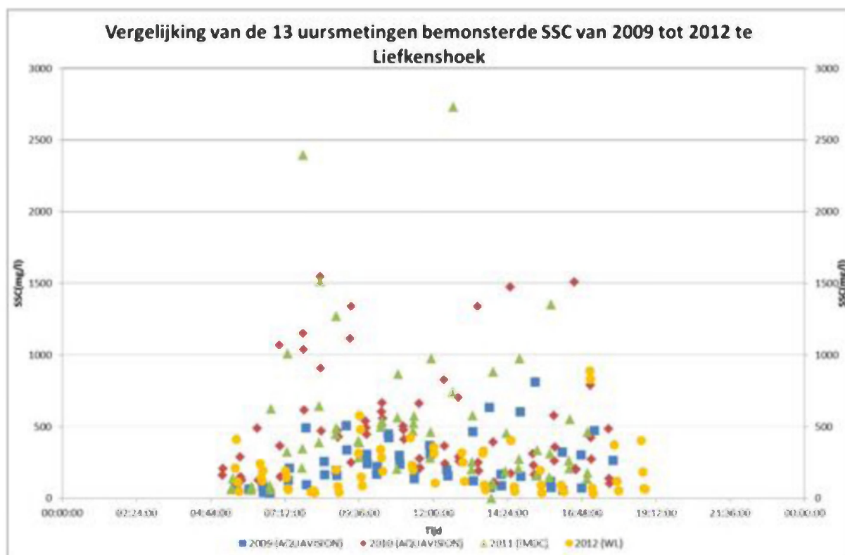
Figuur 147 - Gemeten SSC tijdens de dertienuursmetingen te Liefkenshoek (Beneden-Zeeschelde) in 2009 t.e.m. 2012
