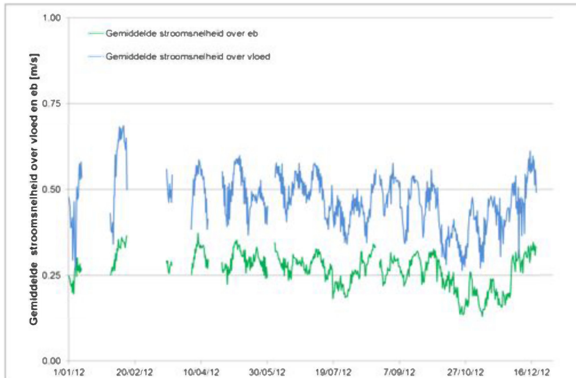
Figuur 56 - Gemiddelde stroomsnelheid over vloed en over eb te Boei 84 (Beneden-Zeeschelde), onderste meettoestel
