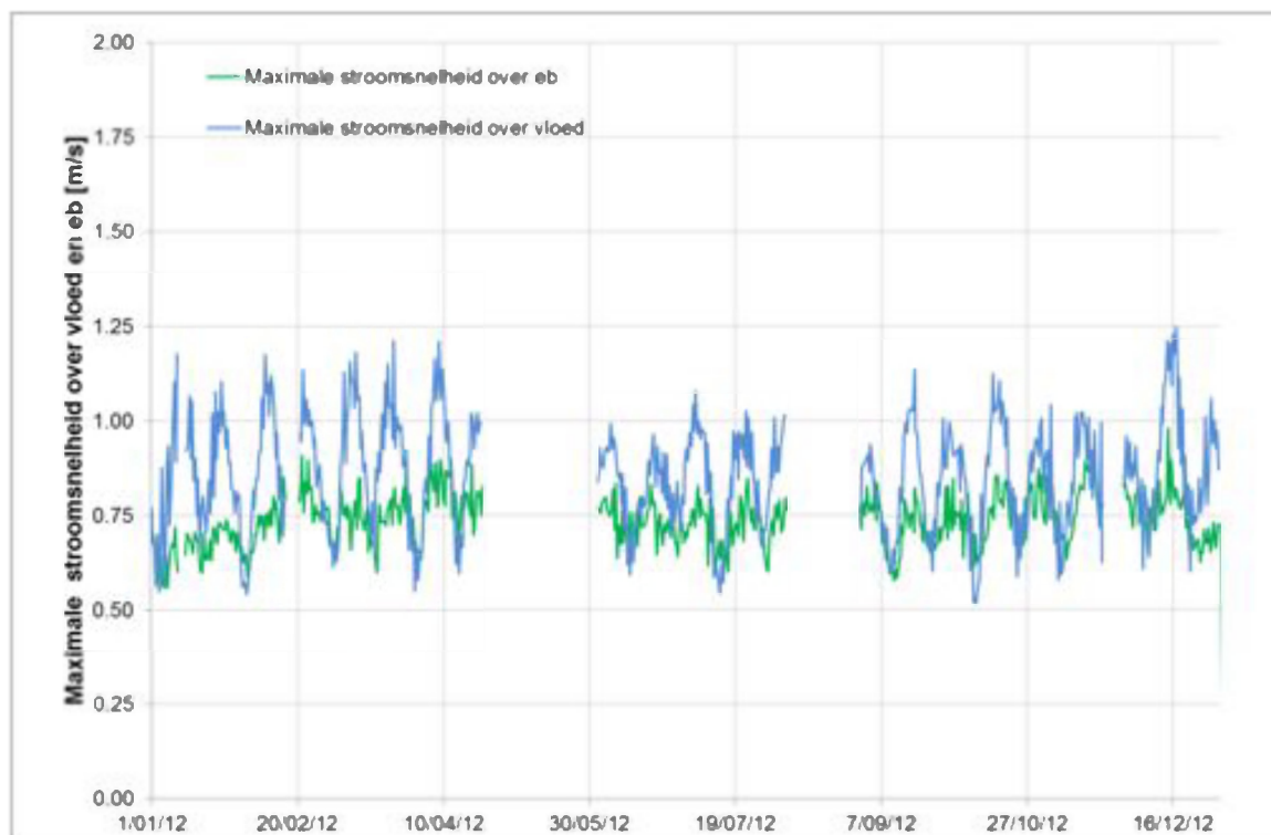
Figuur 63 - Maximale stroomsnelheid over vloed en over eb te Oosterweel (Beneden-Zeeschelde), onderste meettoestel
