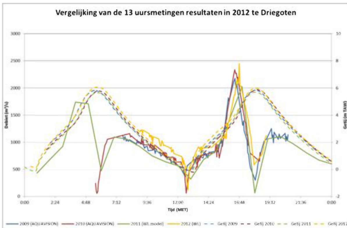
Figuur 159 - Debiet en getij tijdens de dertienuursmetingen te Driegoten (Boven-Zeeschelde) in 2009 t.e.m. 2012
