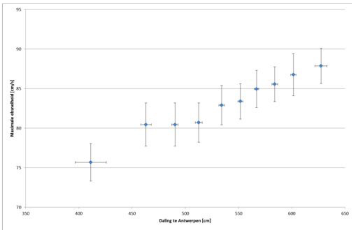
Figuur 74 - Maximale ebsnelheid te Driegoten (Boven-Zeeschelde) versus de daling in waterpeil te Antwerpen
