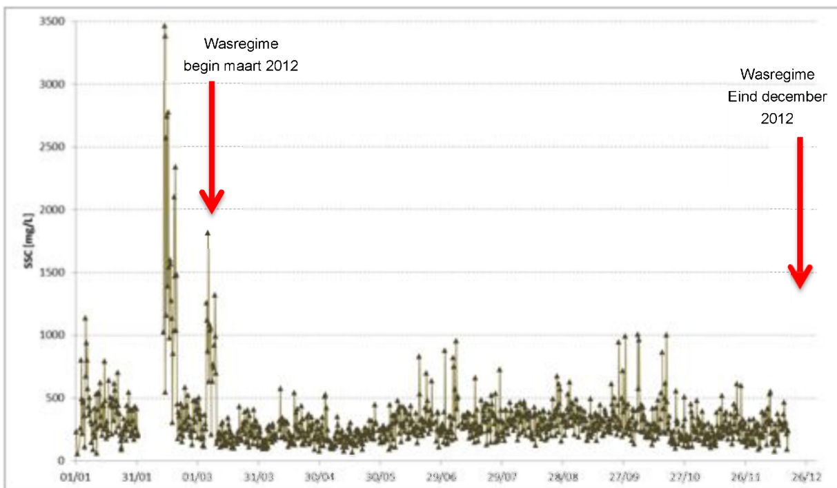
Figuur 127 - SSC (gemeten m.b.v. automatische staalname) te Melle (Boven-Zeeschelde)
