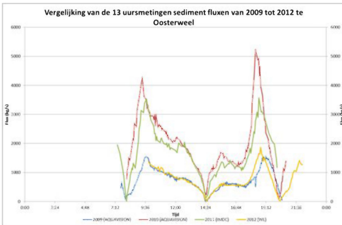
Figuur 153 - SSF tijdens de dertienuursmetingen te Oosterweel (Beneden-Zeeschelde) in 2009 t.e.m. 2012
