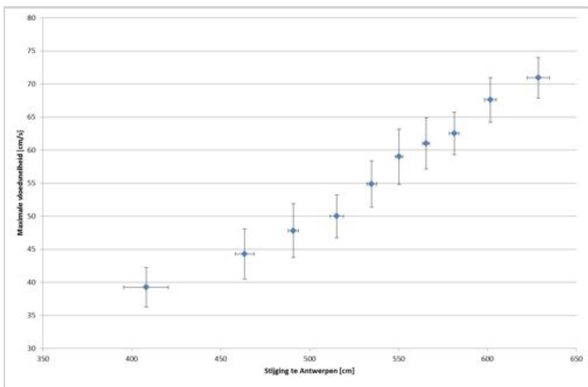
Figuur 75 - Maximale vloed-snelheid te Driegoten (Boven-Zeeschelde) versus de stijging in waterpeil te Antwerpen
