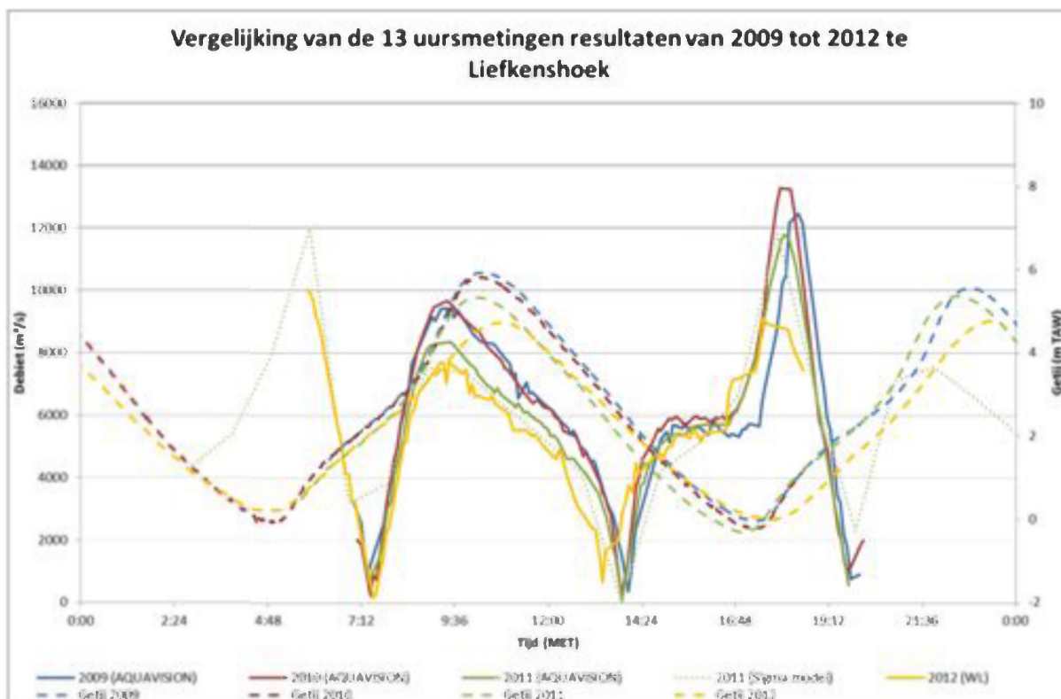
Figuur 146 - Debiet en getij tijdens de dertienuursmetingen te Liefkenshoek (Beneden-Zeeschelde) in 2009 t.e.m. 2012
