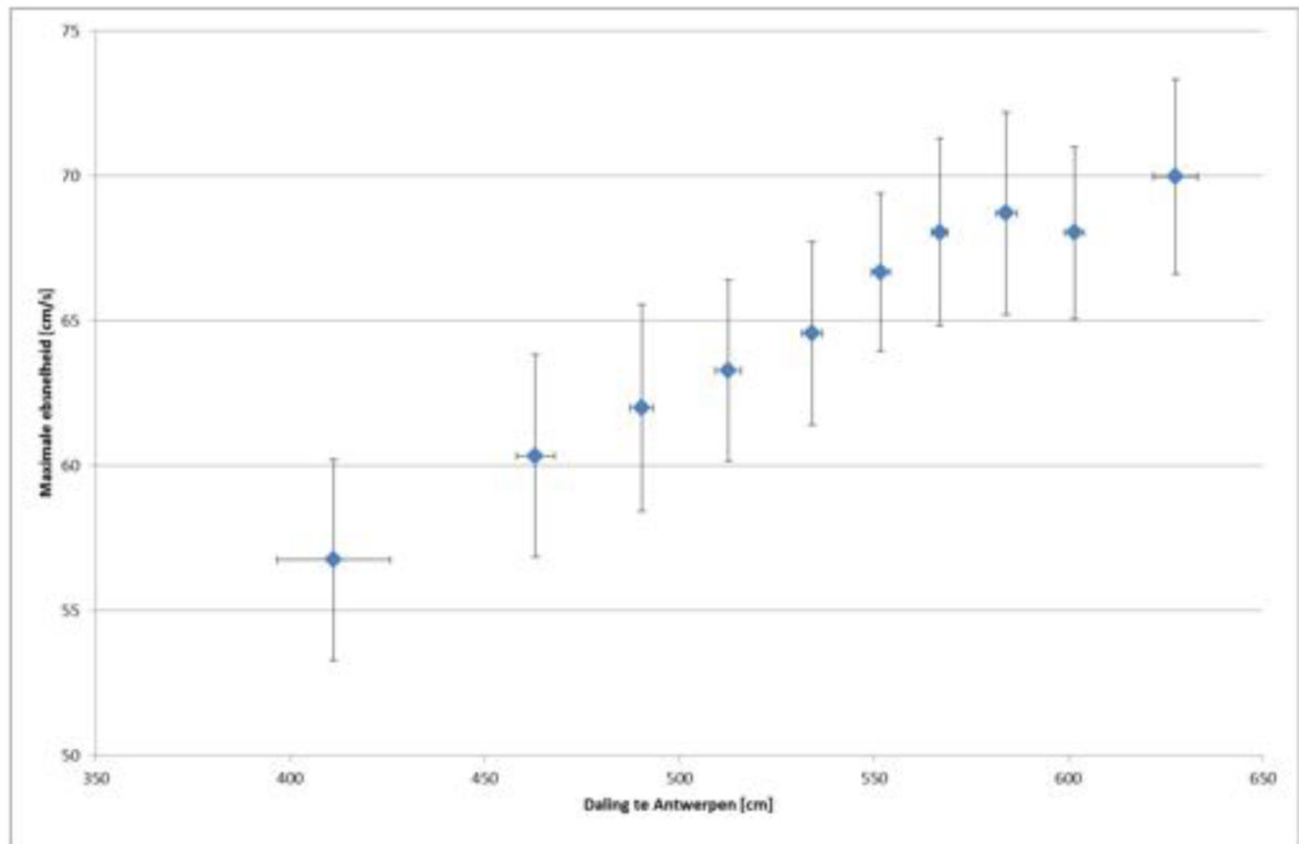
Figuur 66 - Maximale ebsnelheid te Boei 84 (Beneden-Zeeschelde), bovenste meettoestel, versus de daling in waterpeil te Antwerpen
