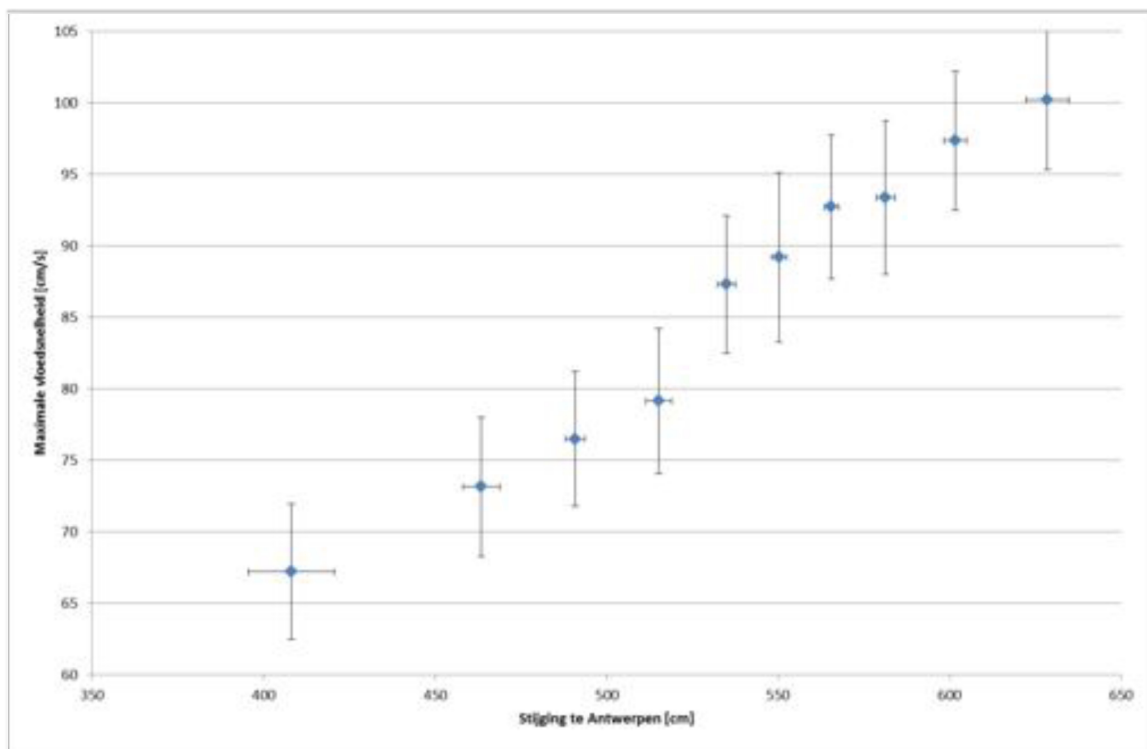
Figuur 73 - Maximale vloednelheid te Oosterweel (Beneden-Zeeschelde), onderste meettoestel, versus de stijging in waterpeil te Antwerpen
