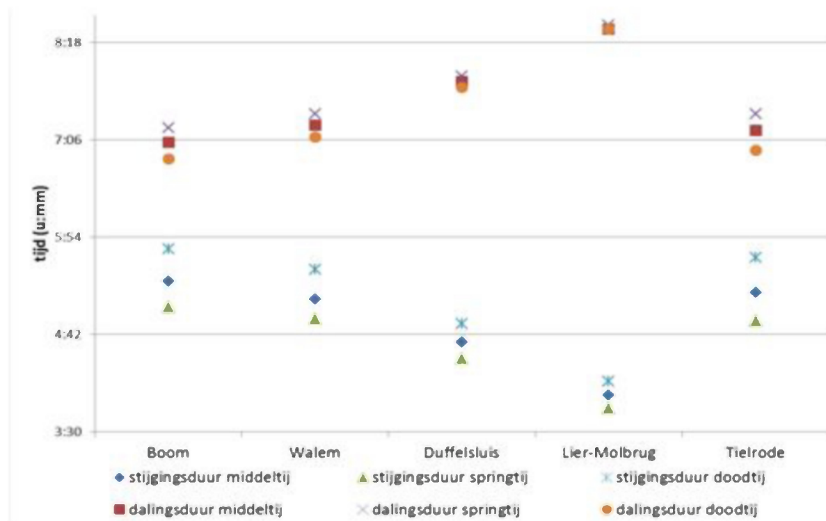
Figuur 13 - Duur van stijging en daling bij middeltij, springtij en doodtij in 2012 voor de Rupel (Boom en Walem), Beneden Nete (Walem en Duffelsluis) en de Durme (Tielrode)
