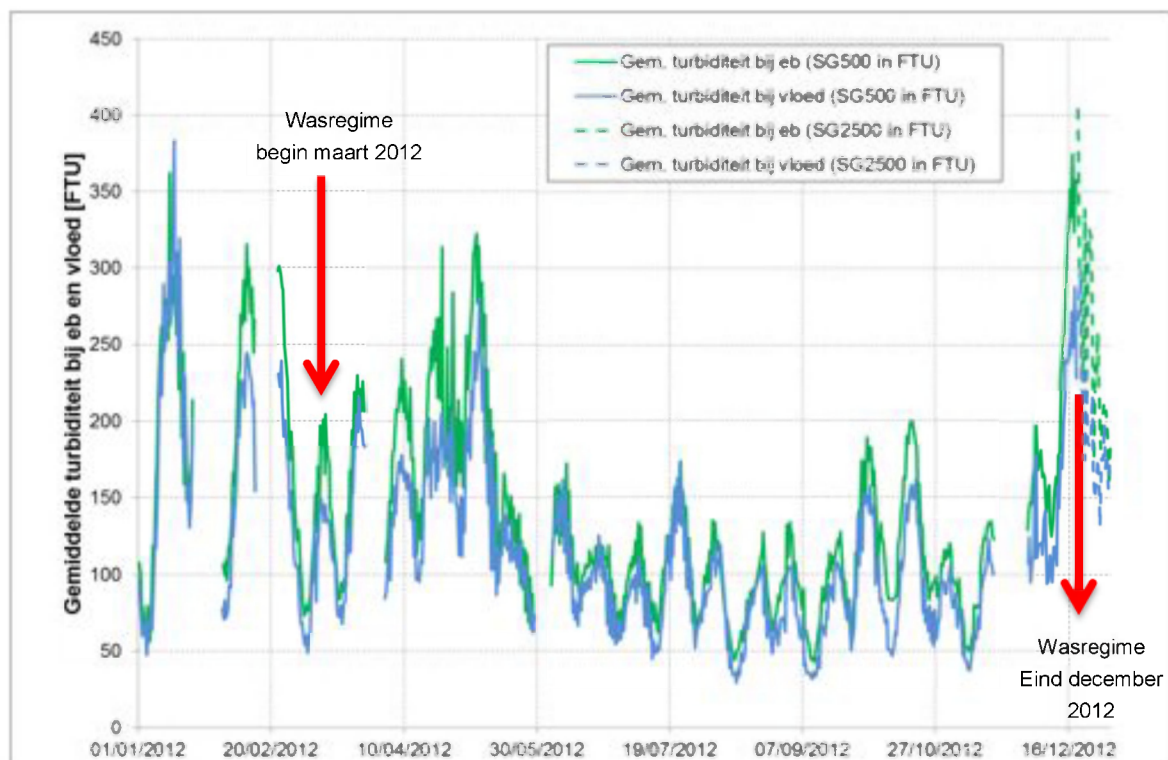
Figuur 98 - Gemiddelde turbiditeit bij eb en vloed te Boei 84 (Beneden-Zeeschelde), bovenste meettoestel
